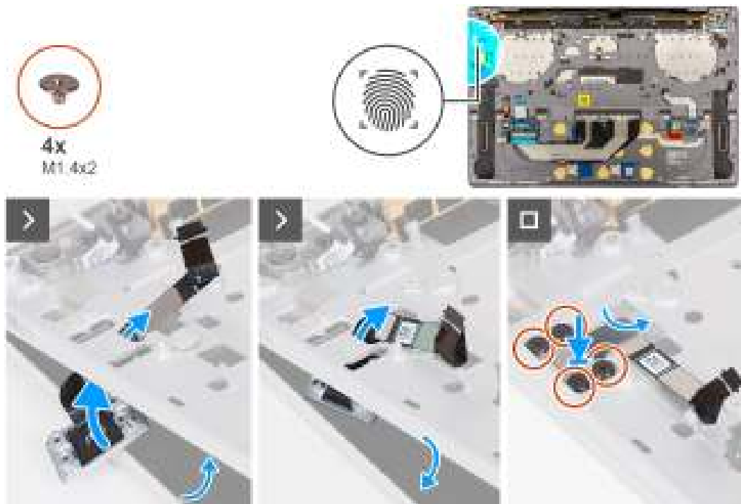
Afbeelding 44. De aan-uitknop met vingerafdruklezer plaatsen
