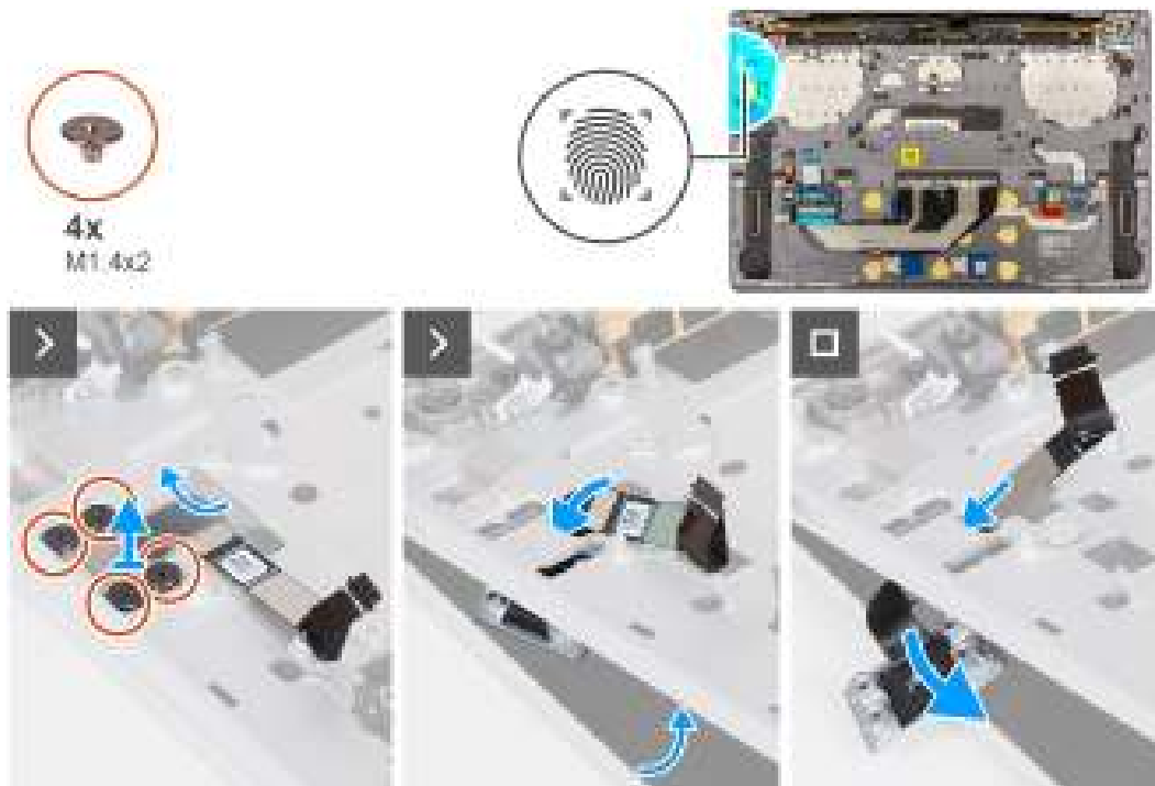
Afbeelding 42. De aan-uitknop met vingerafdrukkezer verwijderen
