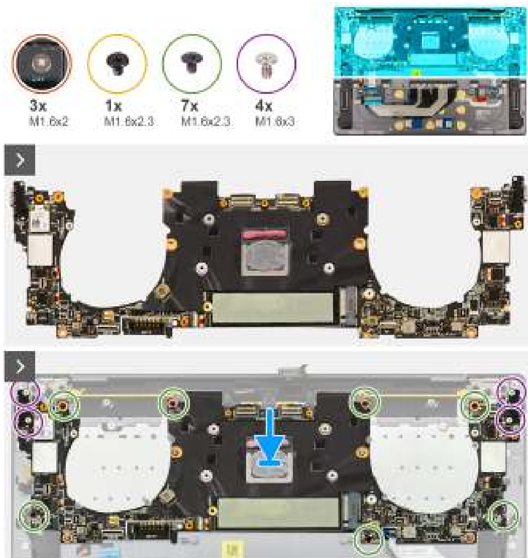
Afbeelding 40. De systeemkaart installeren
