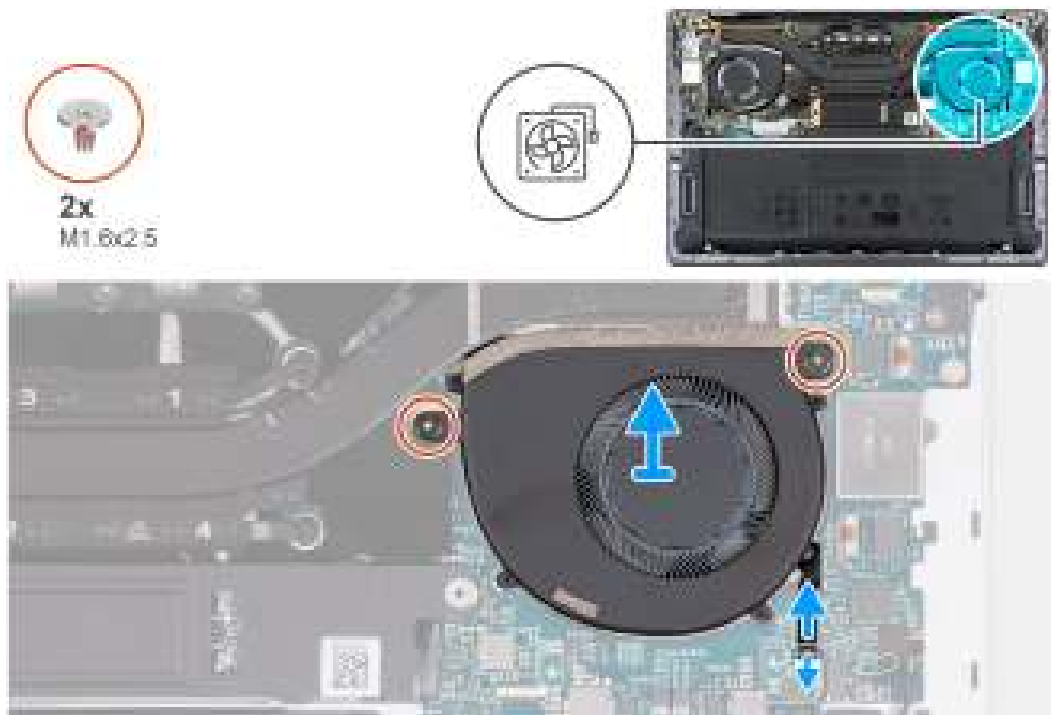
Afbeelding 25. De linkerventilator verwijderen
