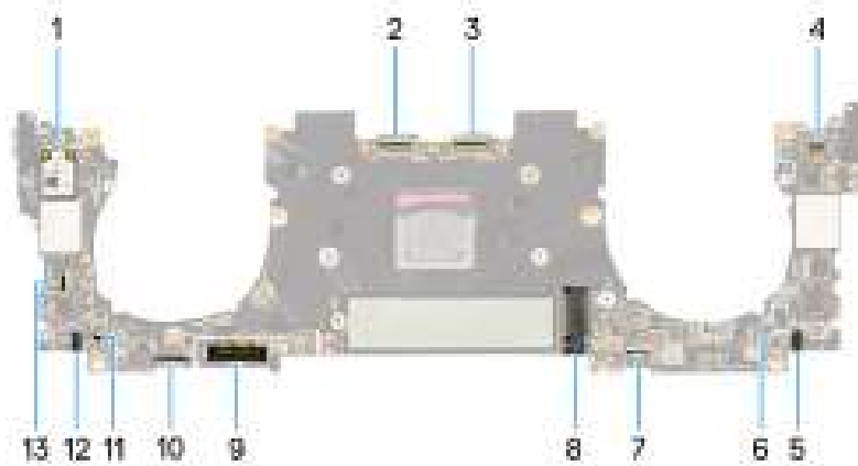
Afbeelding 38. Systeemkaartconnectoren
