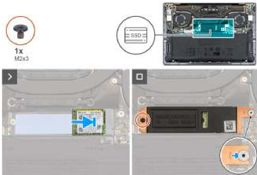
Afbeelding 21. De M.2 2230 SSD plaatsen
