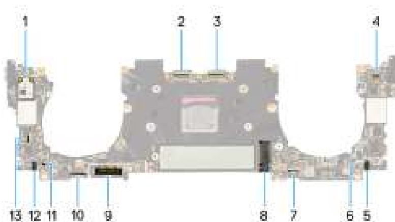
Afbeelding 34. Systeemkaartconnectoren
