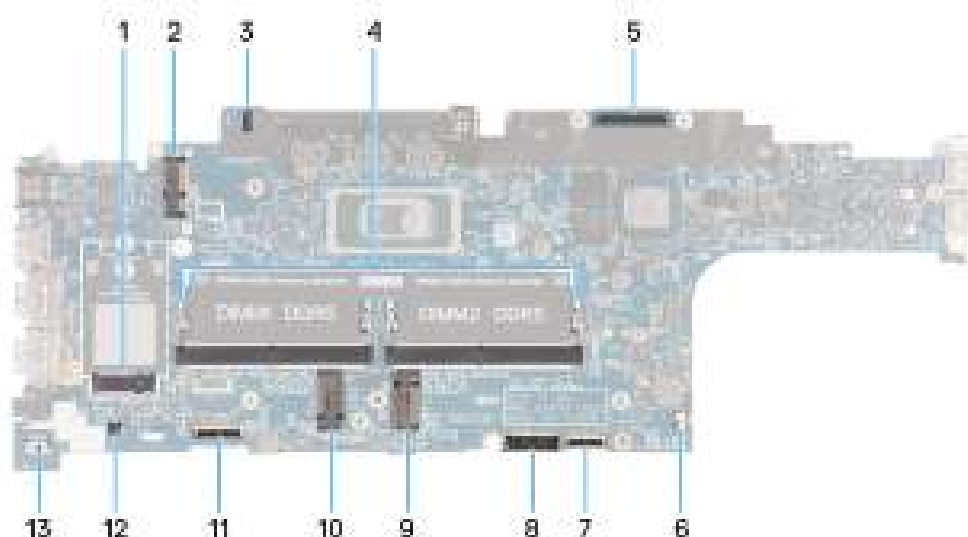
Afbeelding 57. Systeemkaartconnectoren
