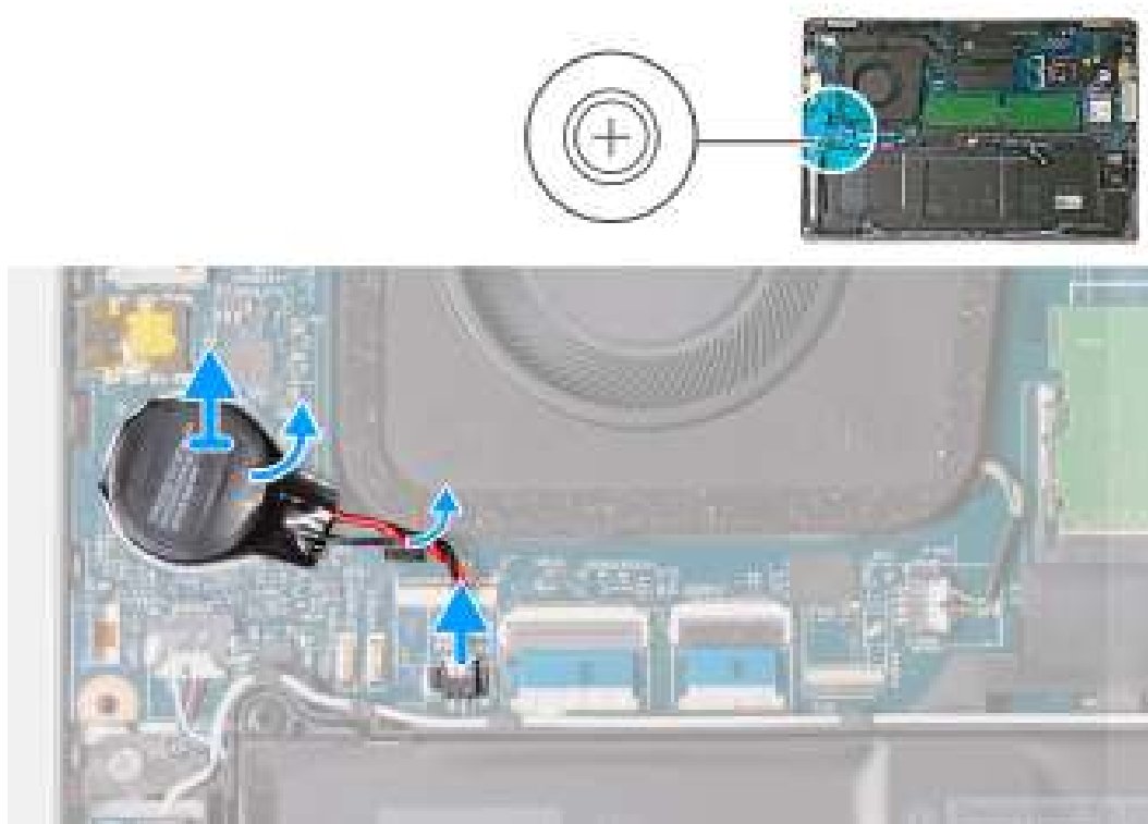
Afbeelding 28. De knoopcelbatterij verwijderen
