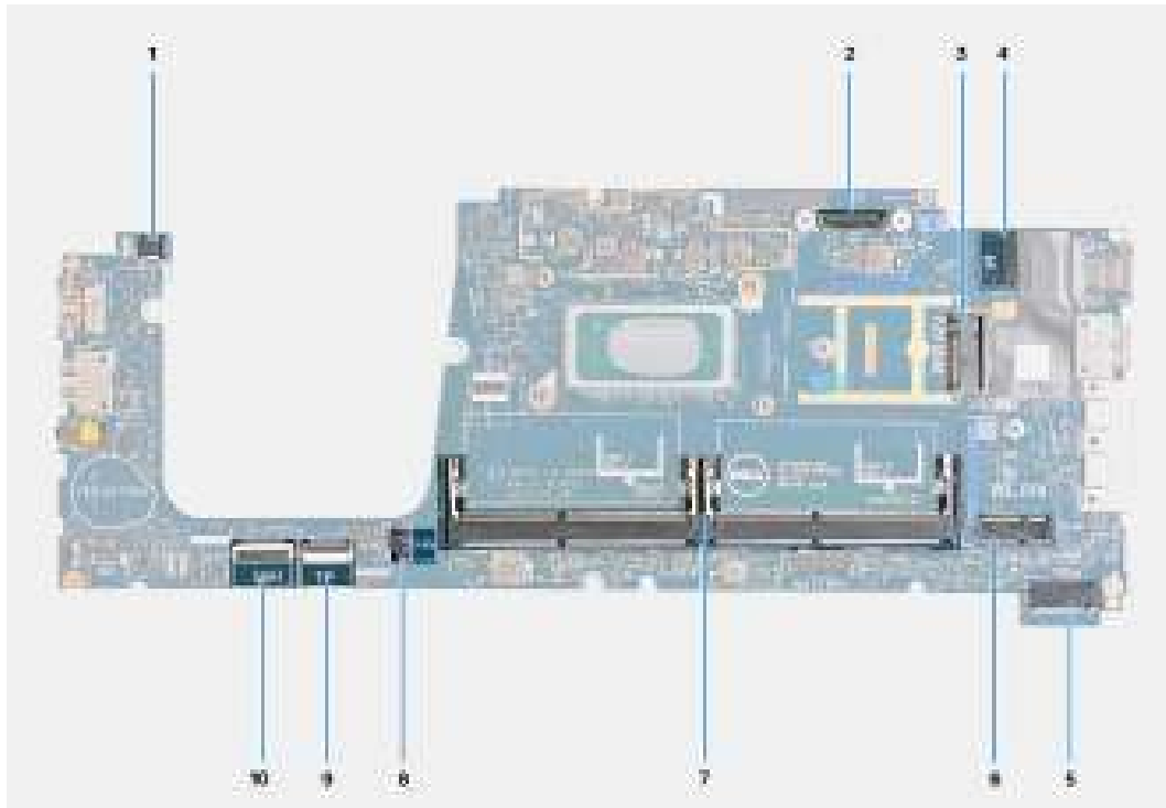
Afbeelding 67. Systeemkaartconnectoren
