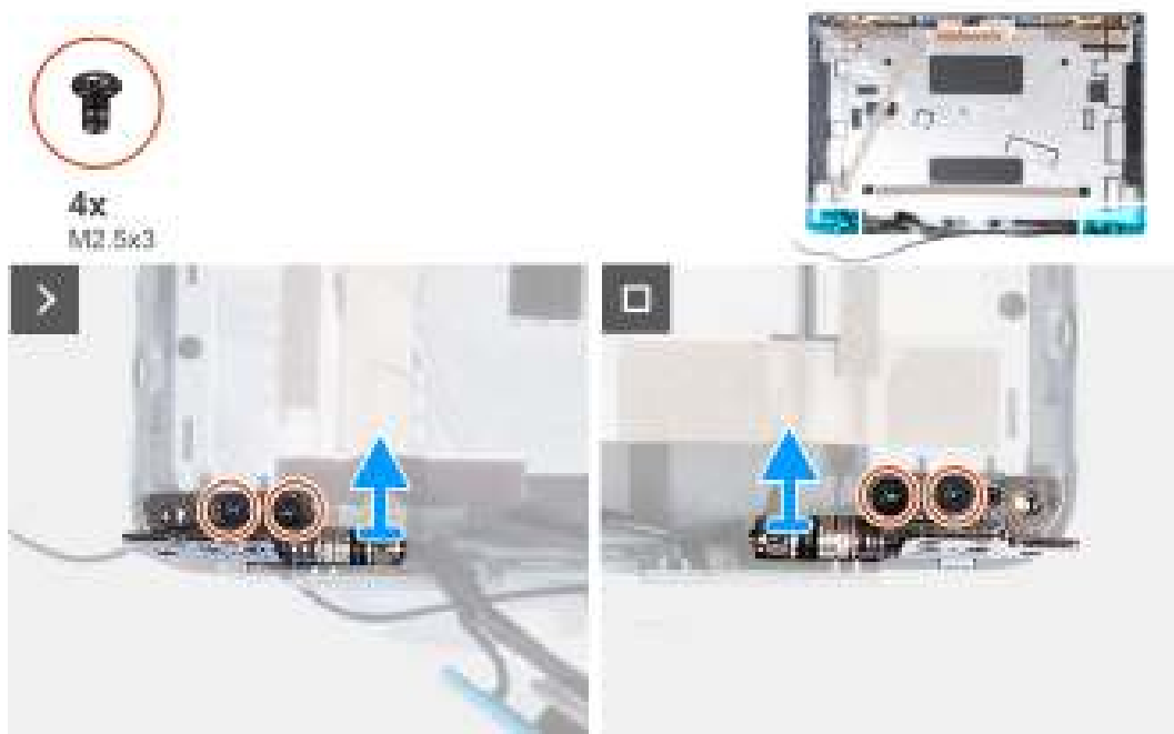
Afbeelding 60. De beeldschermsharnieren verwijderen
