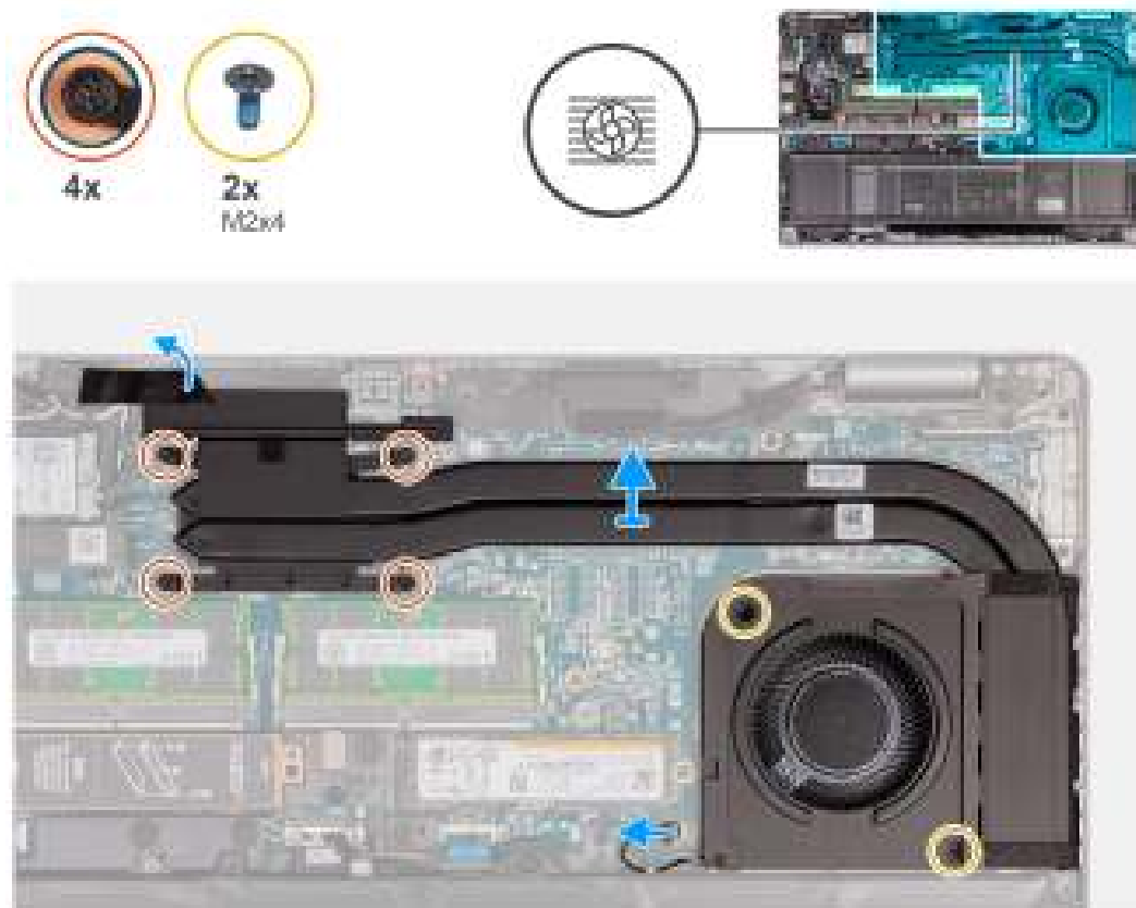
Afbeelding 54. De ventilator- en koelplaateneenheid verwijderen (geïntegreerde GPU)
