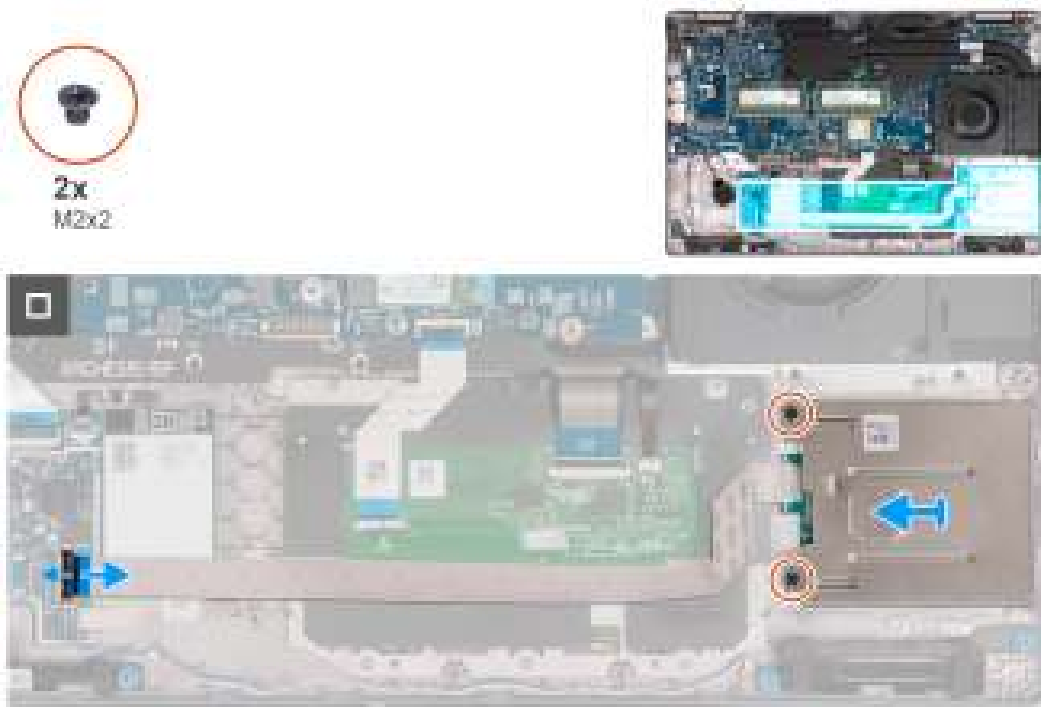
Afbeelding 98. De smartcardlezer verwijderen
