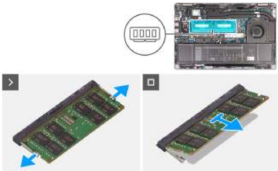
Afbeelding 25. De geheugenmodule verwijderen
