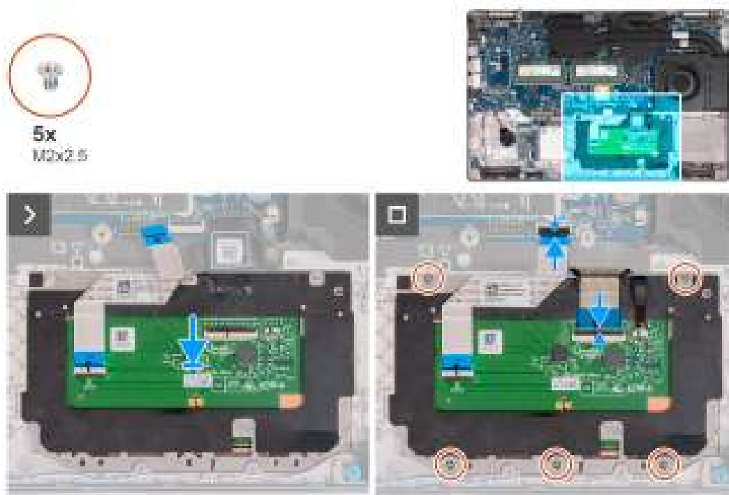
Afbeelding 46. De touchpad installeren
