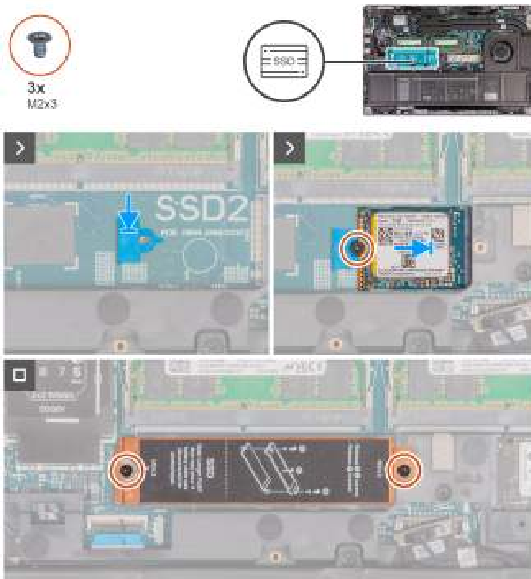
Afbeelding 32. De M.2 2230 SSD in slot 2 installeren
