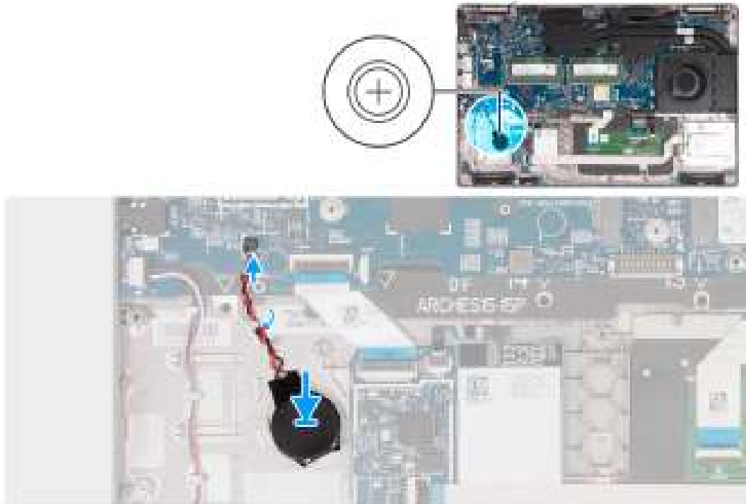
Afbeelding 51. De knoopcelbatterij plaatsen
