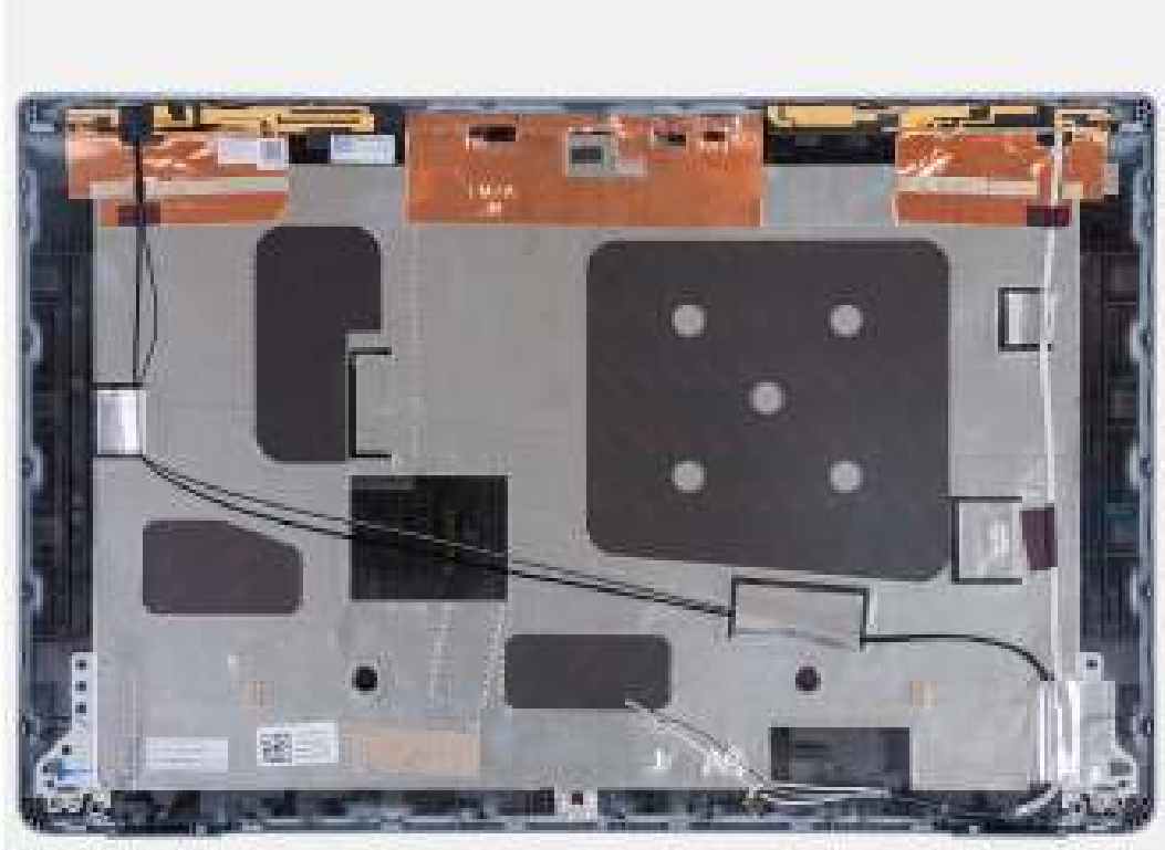
Afbeelding 93. Het achterpaneel van het beeldscherm installeren
