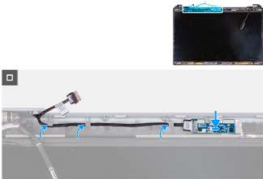
Afbeelding 97. De sensorkaart plaatsen
