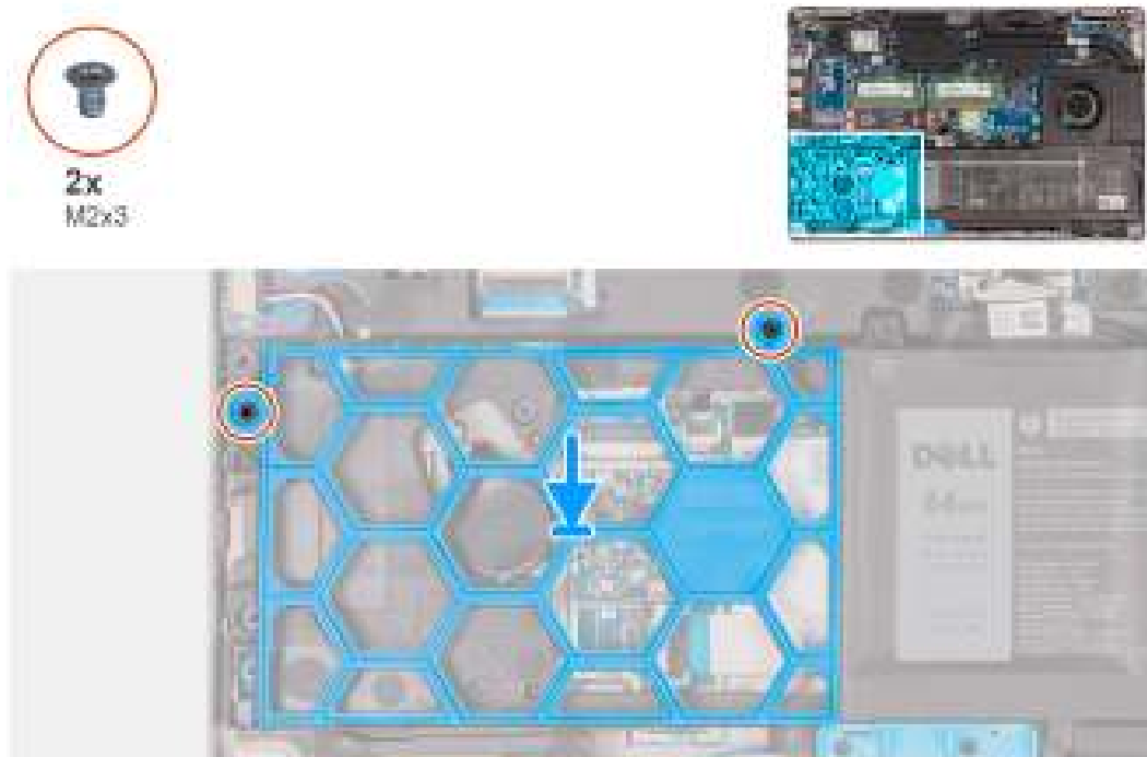
Afbeelding 36. Het plastic inzetstuk installeren
