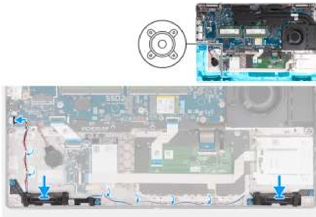
Afbeelding 48. De luidsprekers installeren
