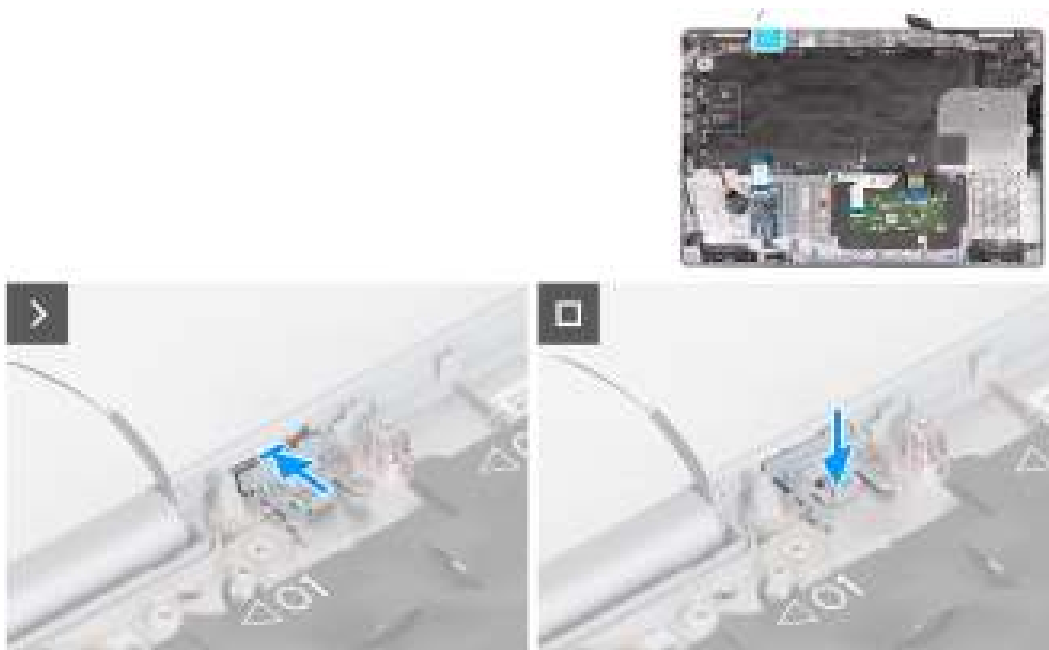
Afbeelding 101. De dummy simkaartslotvuller installeren
