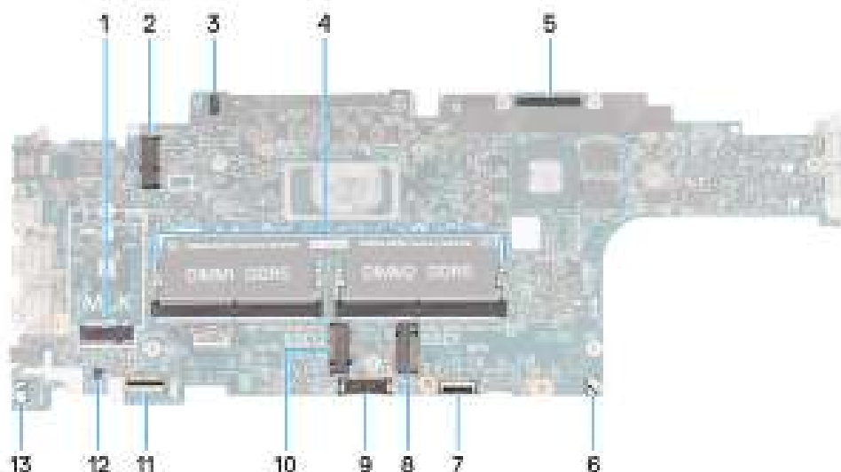
Afbeelding 61. Systeemkaartconnectoren
