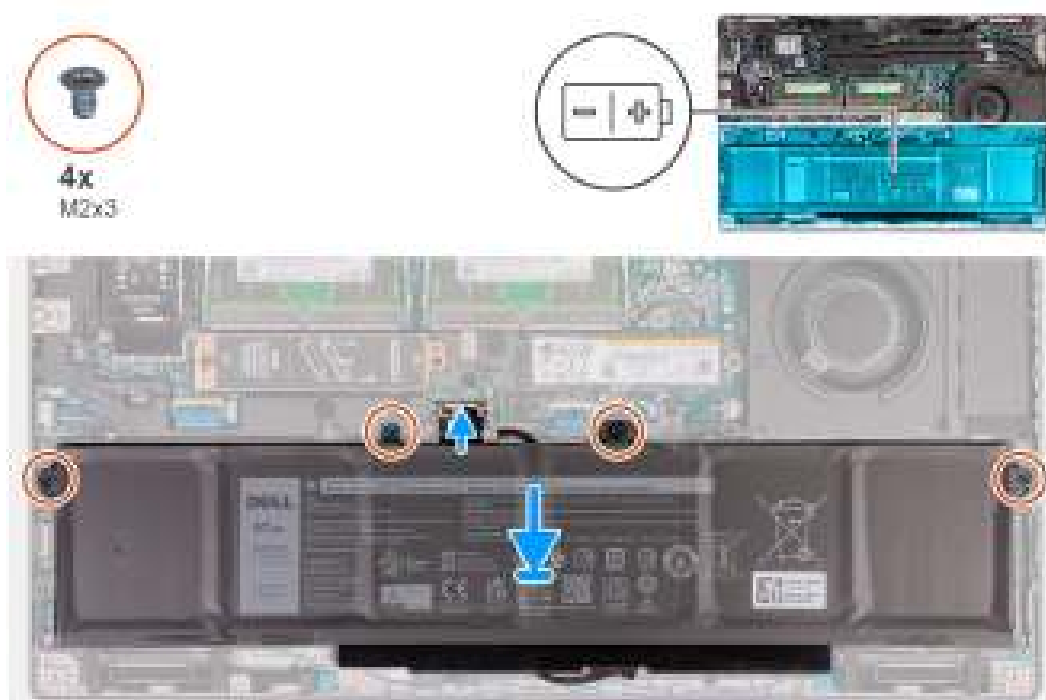
Afbeelding 40. De 97 Whr batterij installeren
