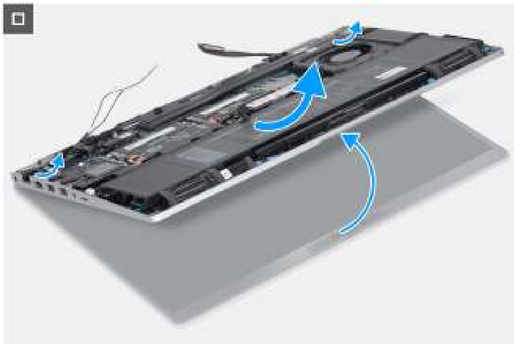
Afbeelding 74. De beeldschermeenheid verwijderen
