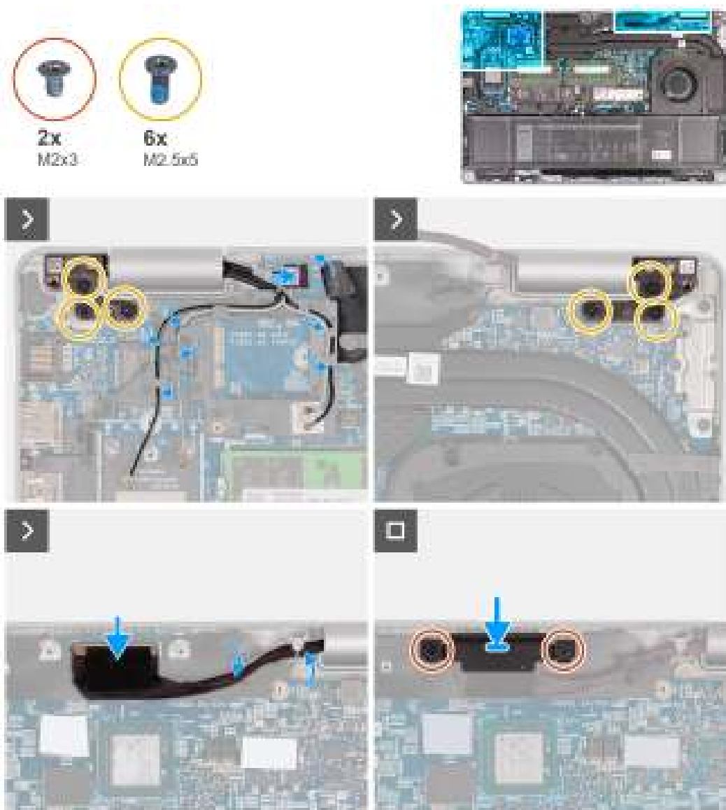
Afbeelding 77. De beeldschermenheid plaatsen
