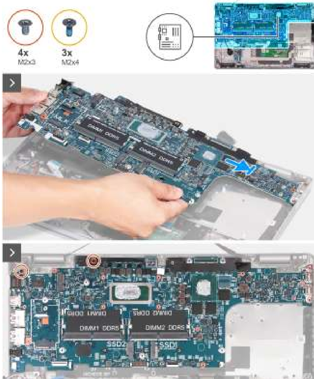
Afbeelding 62. De systeemkaart installeren
