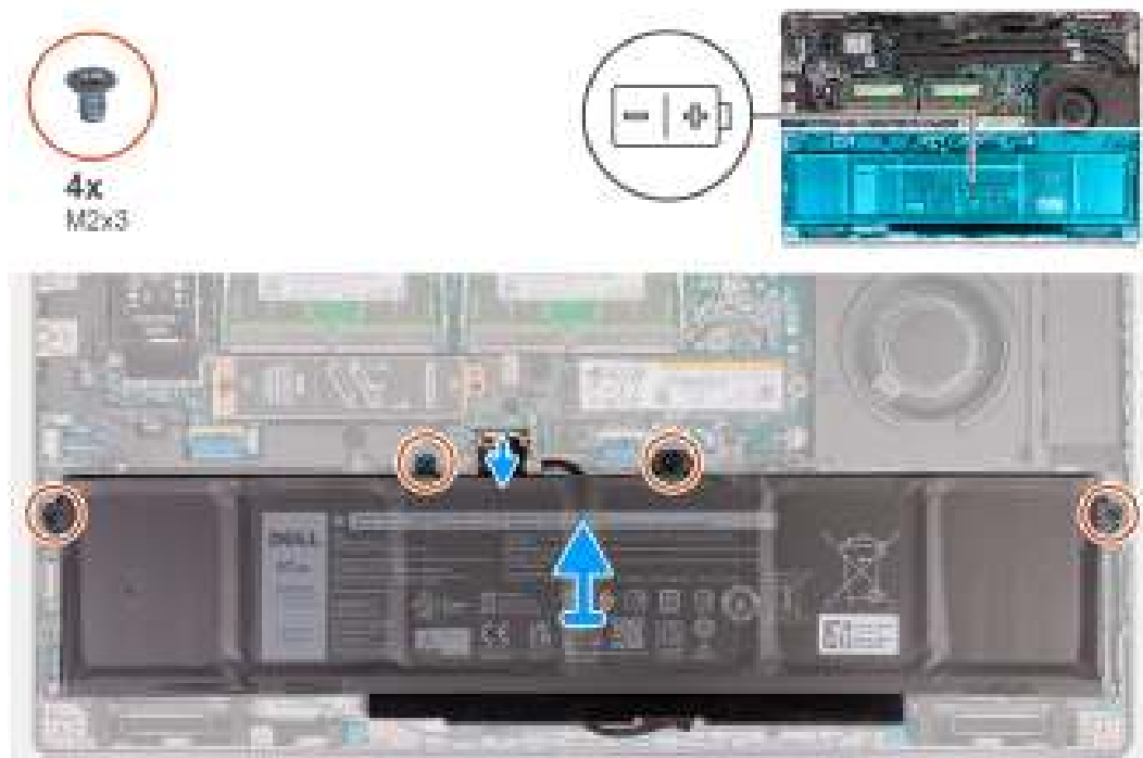
Afbeelding 38. De batterij verwijderen - 97 Whr
