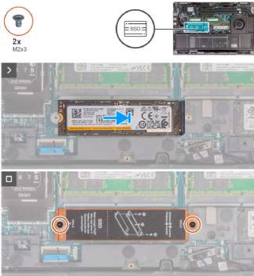
Afbeelding 34. De M.2 2280 SSD in slot 2 installeren
