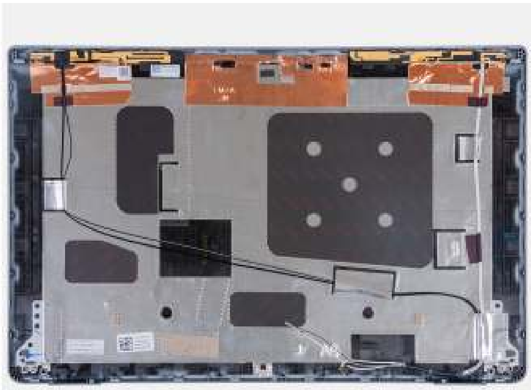
Afbeelding 92. Het achterpaneel van het beeldscherm verwijderen
