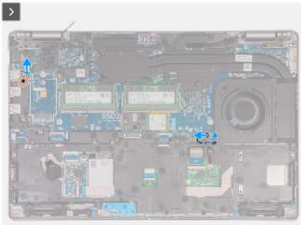
Afbeelding 41. Het binnenframe van de eenheid verwijderen
