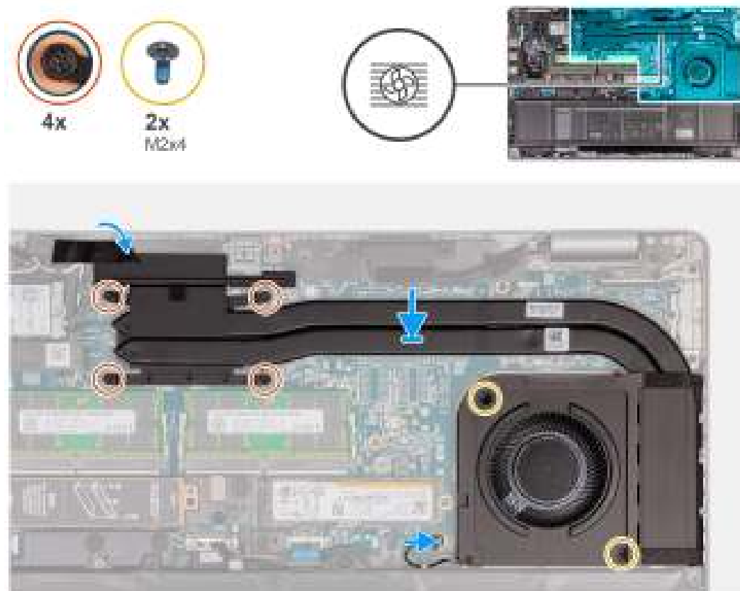
Afbeelding 55. De ventilator- en koelplaateneheid plaatsen (geïntegreerde GPU)
