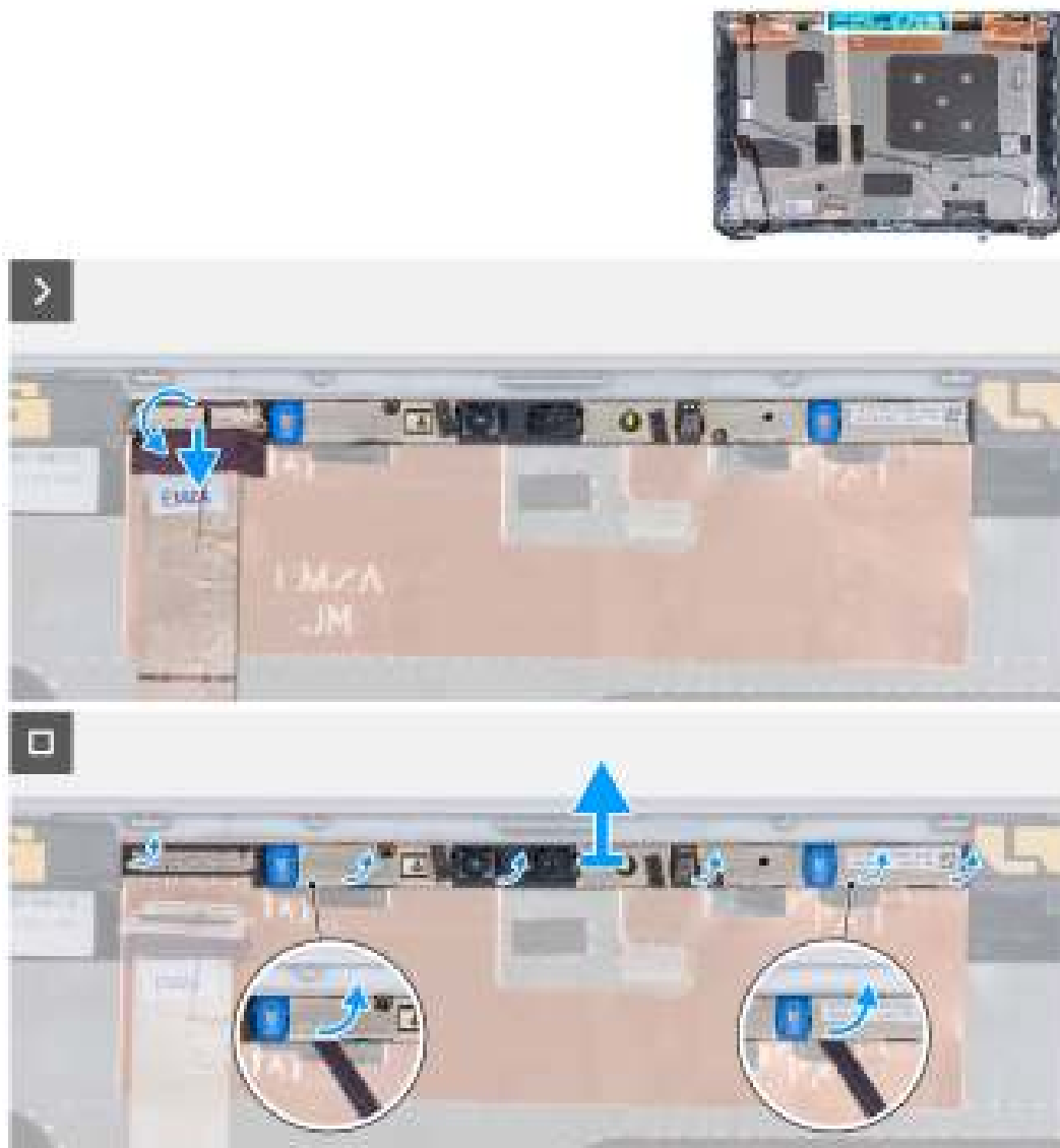
Afbeelding 88. De cameramodule verwijderen
