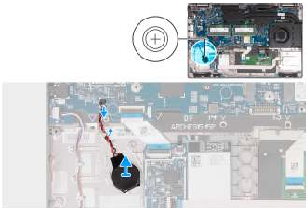
Afbeelding 50. De knoopcelbatterij verwijderen
