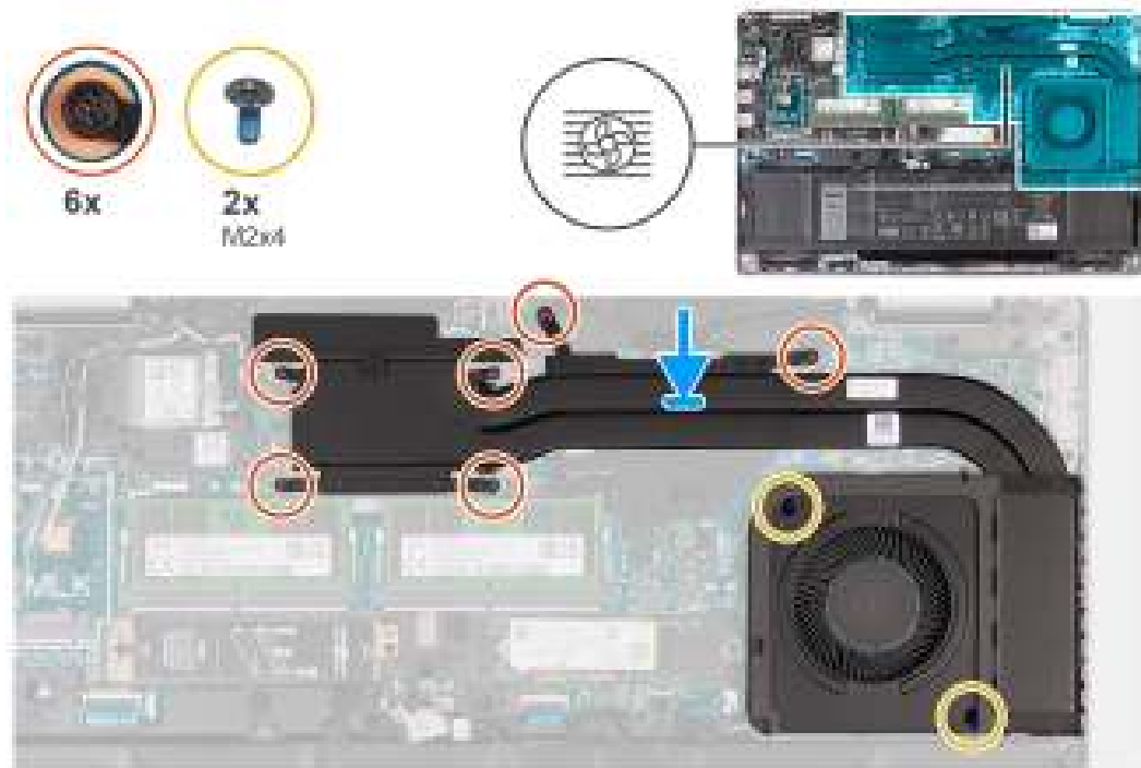
Afbeelding 53. De koelplaat plaatsen (afzonderlijke GPU)
