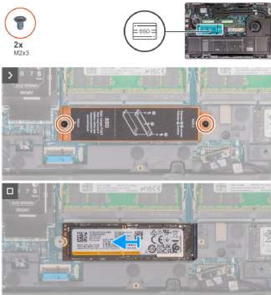
Afbeelding 33. De M.2 2280 SSD verwijderen uit slot 2
