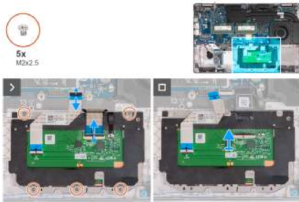
Afbeelding 45. De touchpad verwijderen
