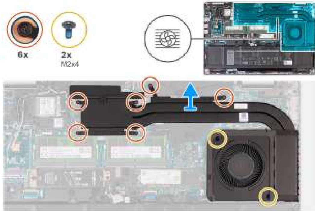
Afbeelding 52. De koelplaat verwijderen (voor afzonderlijke GPU)
