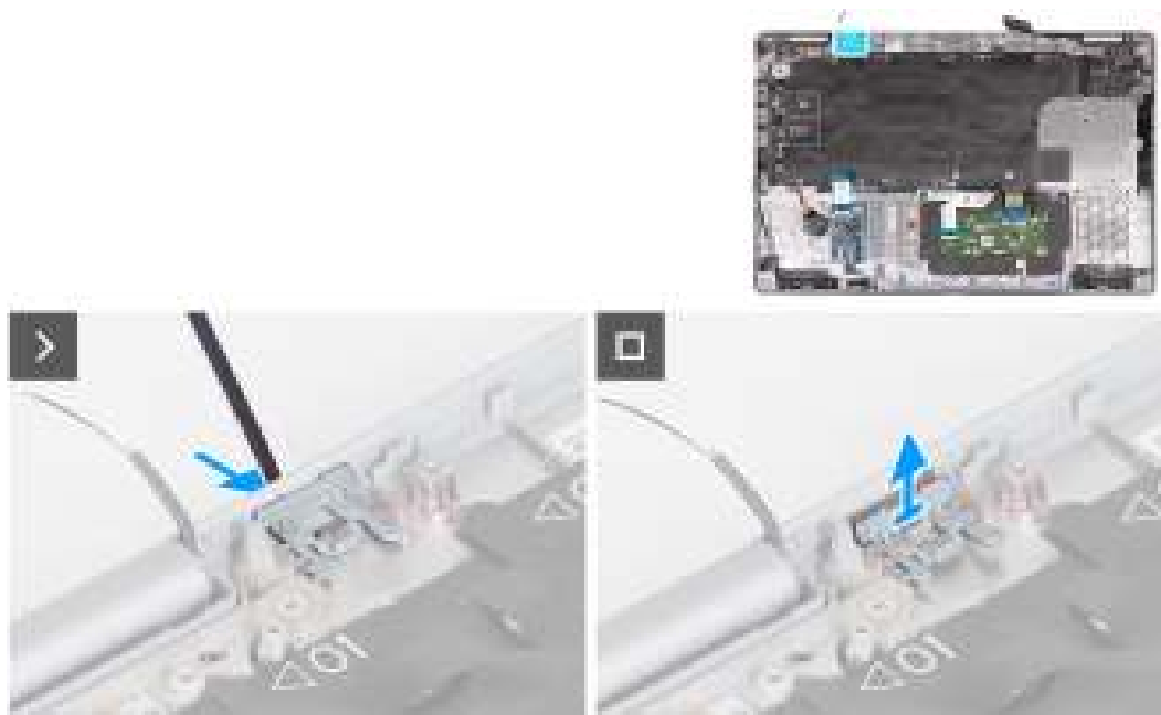
Afbeelding 100. De dummy simkaartslotvuller verwijderen
