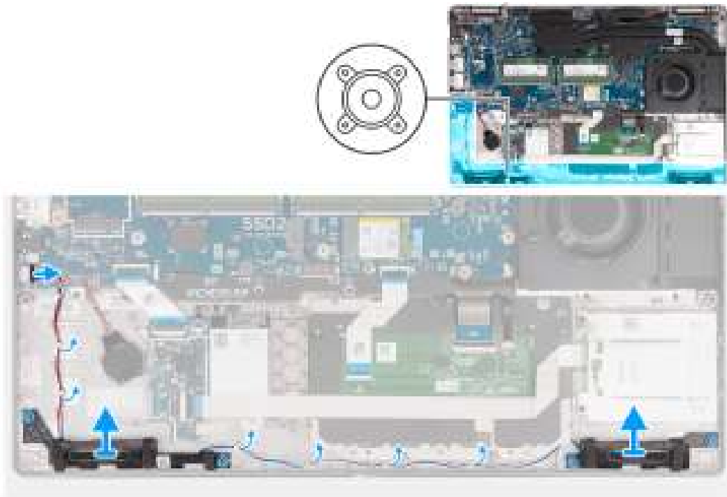
Afbeelding 47. De luidsprekers verwijderen
