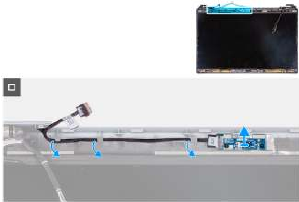
Afbeelding 96. De sensorkaart verwijderen
