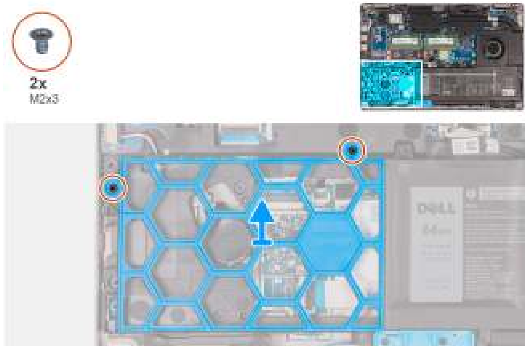
Afbeelding 35. Het plastic inzetstuk verwijderen
