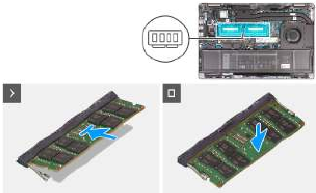
Afbeelding 26. De geheugenmodule plaatsen
