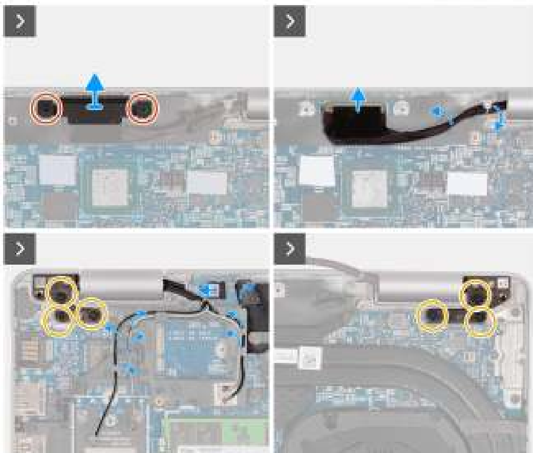
Afbeelding 73. De beeldscherm eenheid verwijderen
