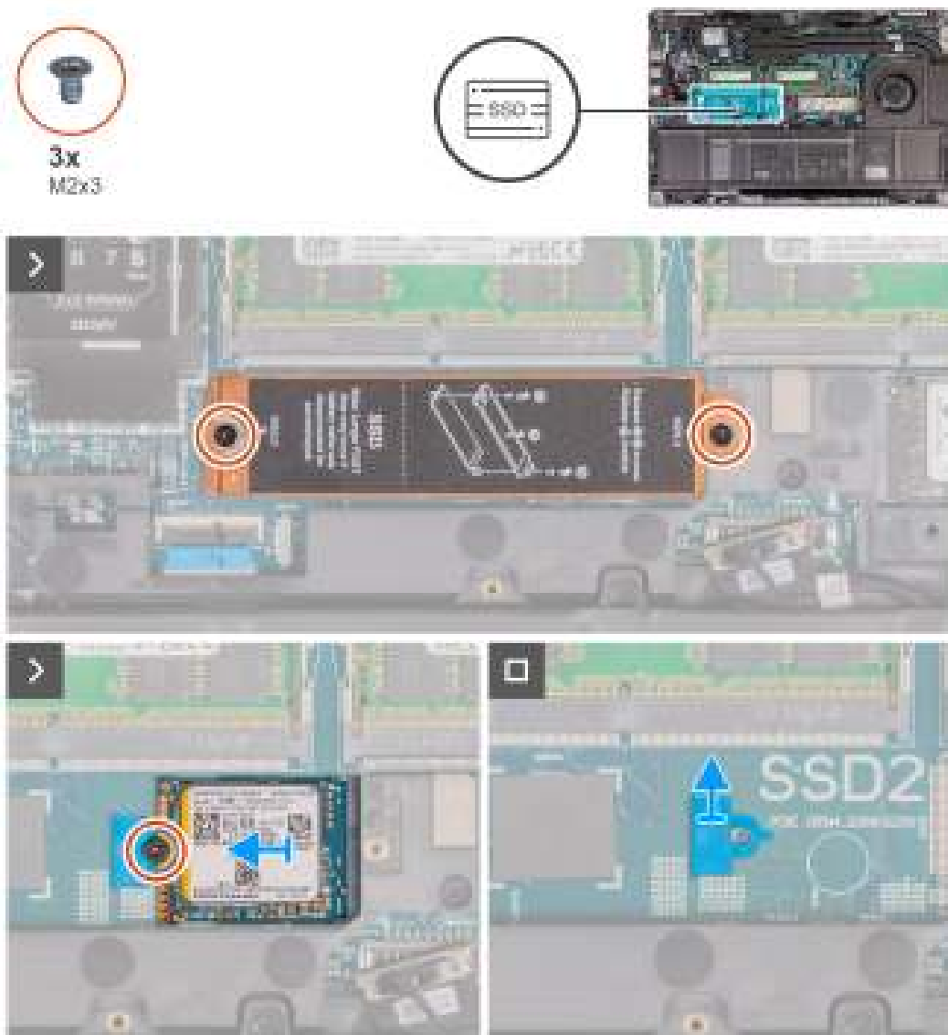
Afbeelding 31. De M.2 2230 SSD verwijderen uit slot 2
