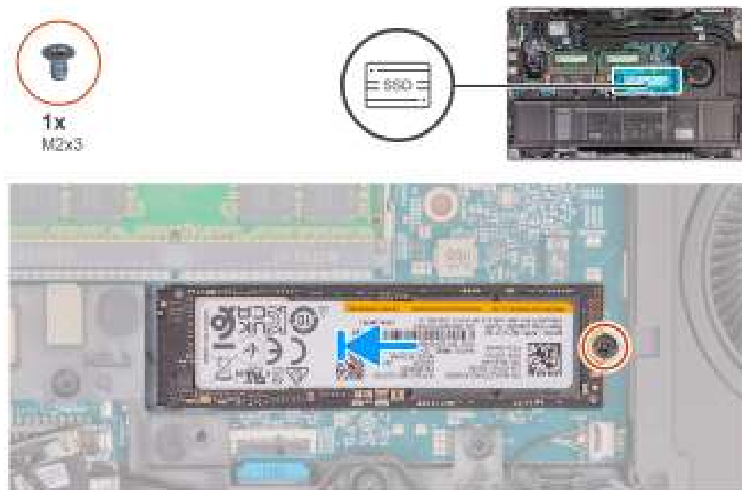
Afbeelding 30. De M.2 2280 SSD in slot 1 installeren
