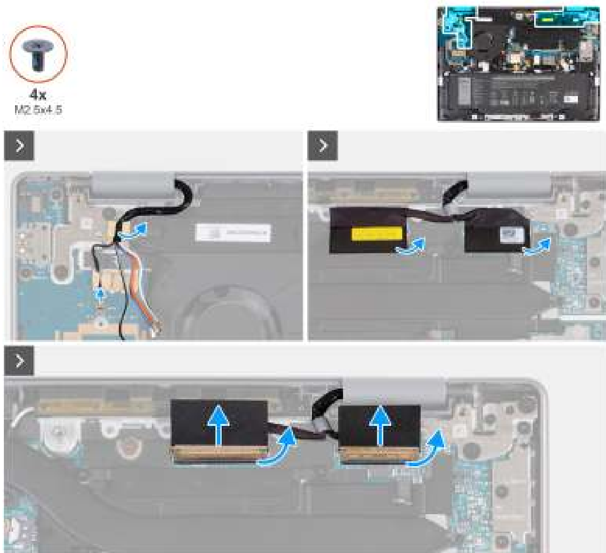
Afbeelding 77. De beeldschermeenheid verwijderen (voor computers die worden geleverd met WWAN-ondersteuning)
