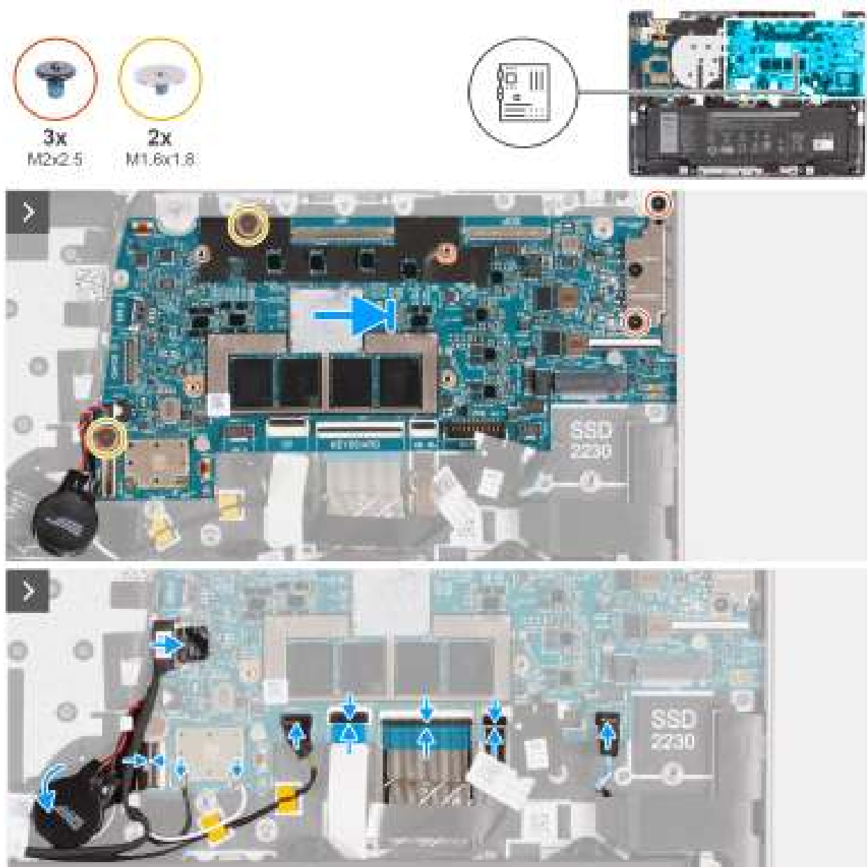
Afbeelding 98. De systeemkaart plaatsen
