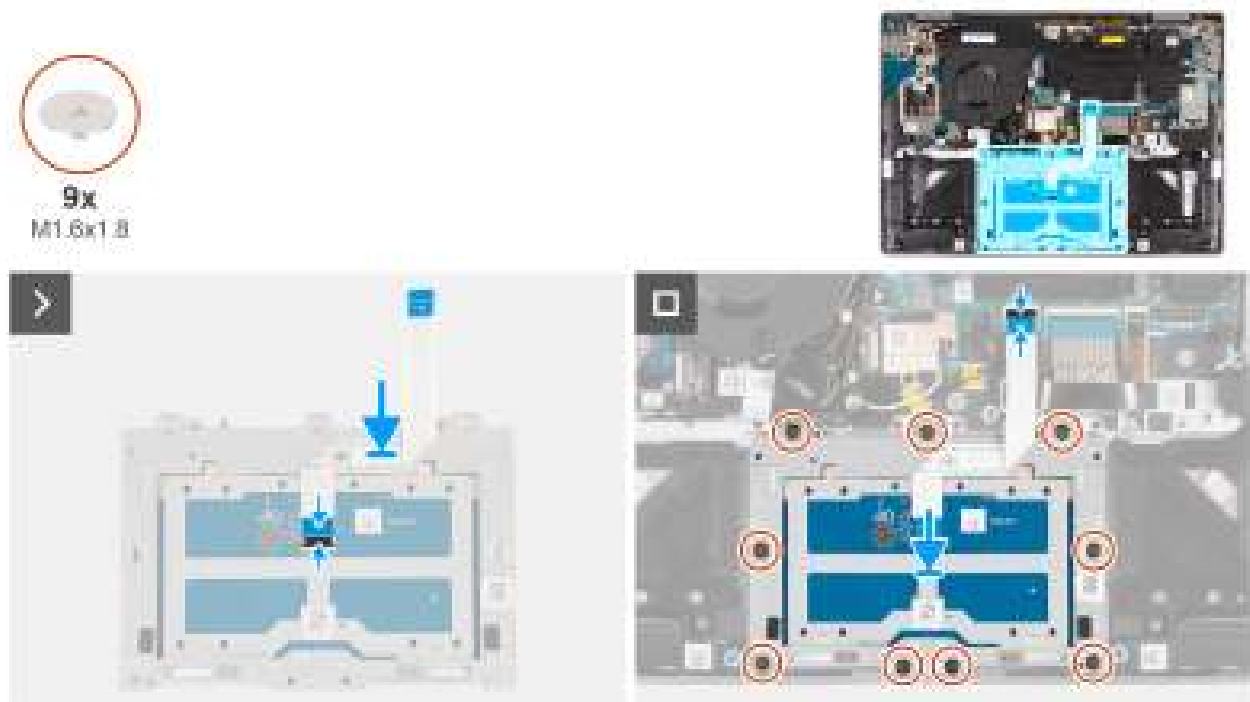
Afbeelding 87. De touchpadeenheid plaatsen
