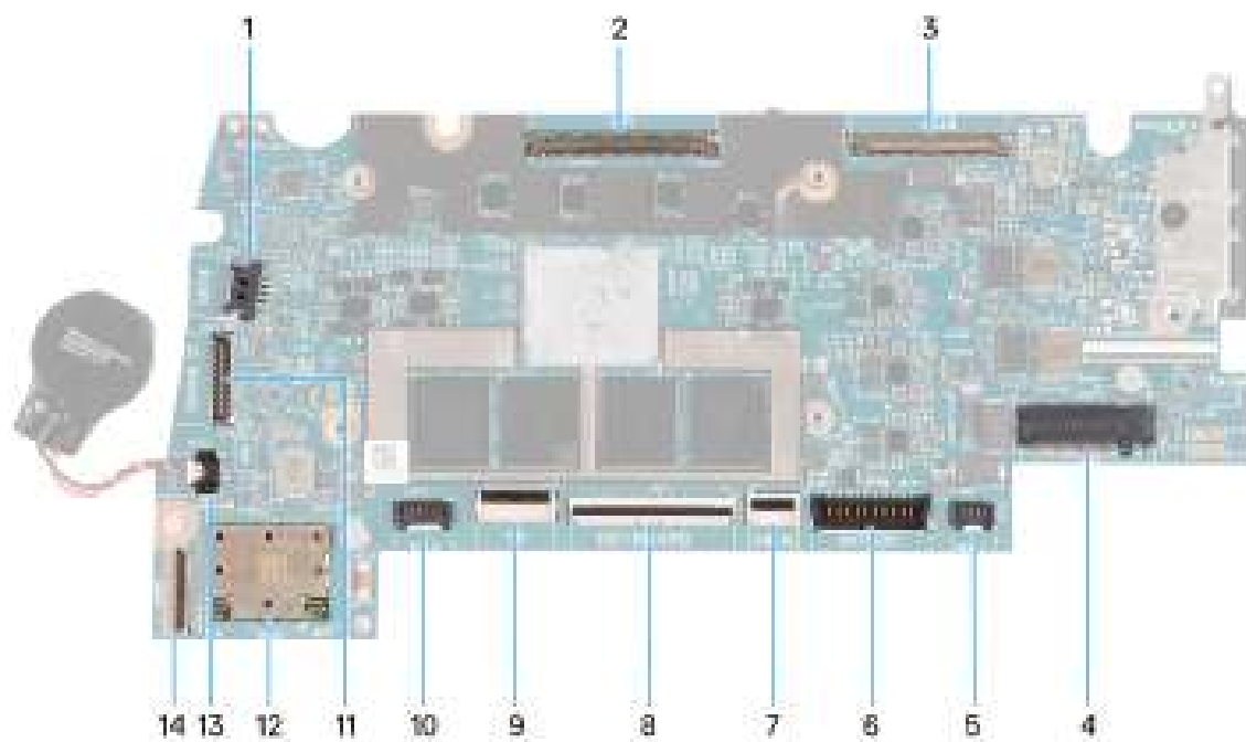
Afbeelding 93. Systeemkaartconnectoren
