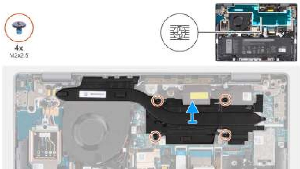
Afbeelding 44. De koelplaat verwijderen
