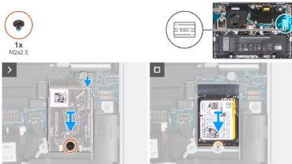
Afbeelding 21. De SSD verwijderen
