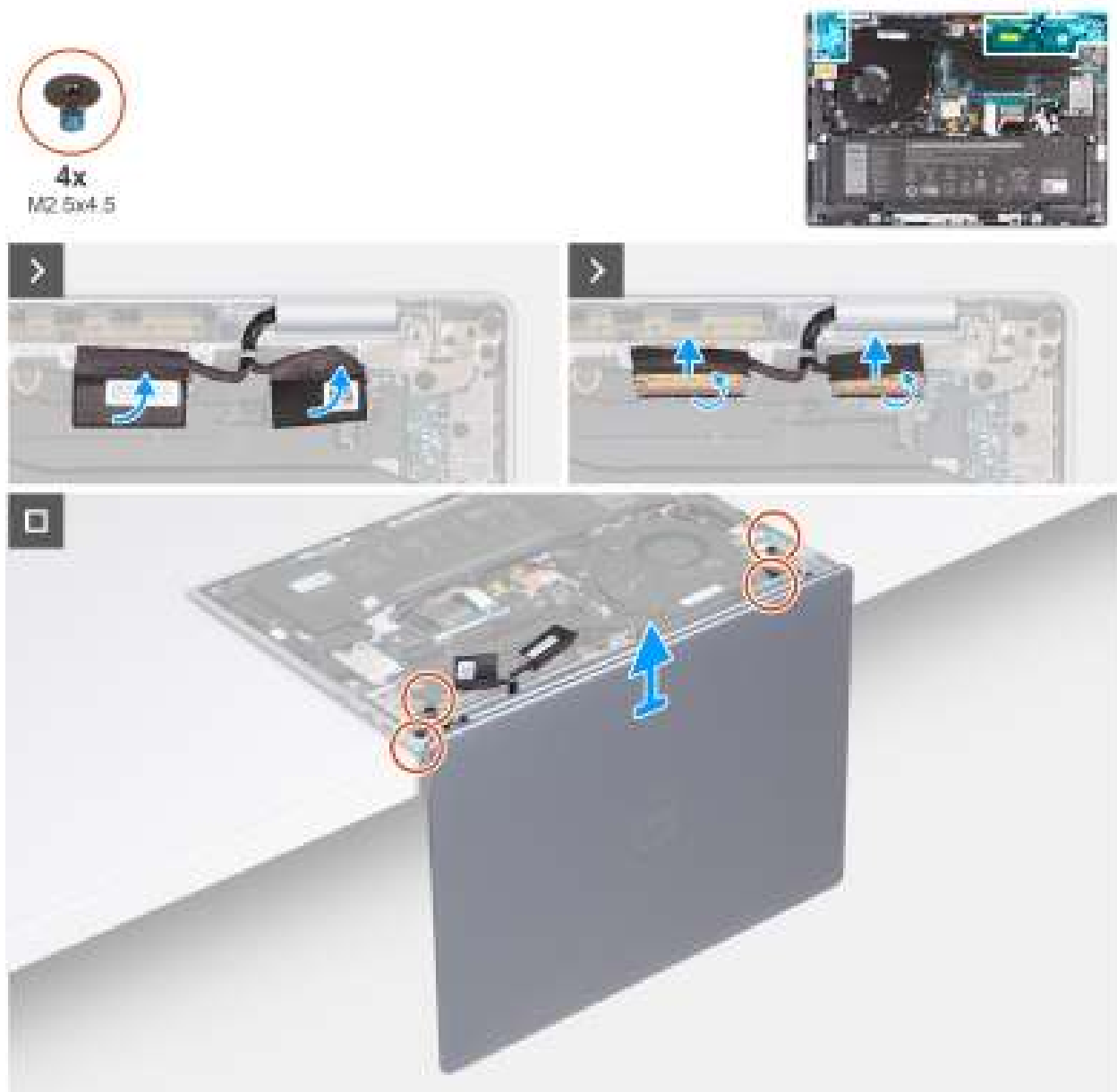
Afbeelding 74. De beeldschermeenheid verwijderen (voor computers die worden geleverd met alleen WLAN-ondersteuning)
