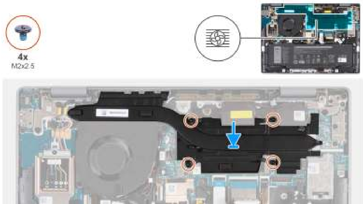
Afbeelding 45. De koelplaat plaatsen
