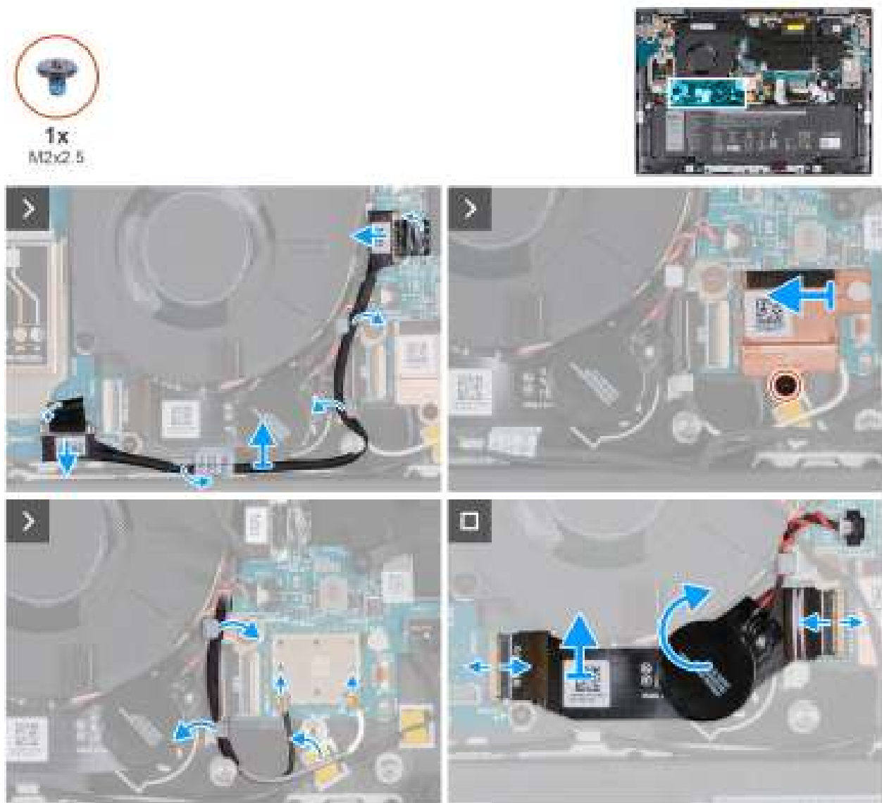
Afbeelding 56. De FPC-kabel van de I/O-kaart verwijderen
