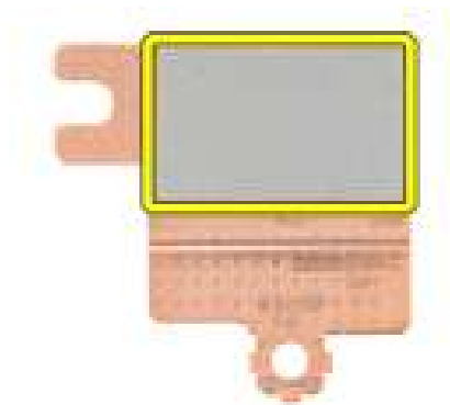
Afbeelding 72. Thermische pad onder het thermische schild van de WLAN-kaart
