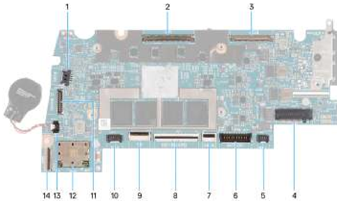
Afbeelding 97. Systeemkaartconnectoren
