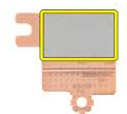
Afbeelding 63. Thermische pad onder het thermische schild van de WLAN-kaart
