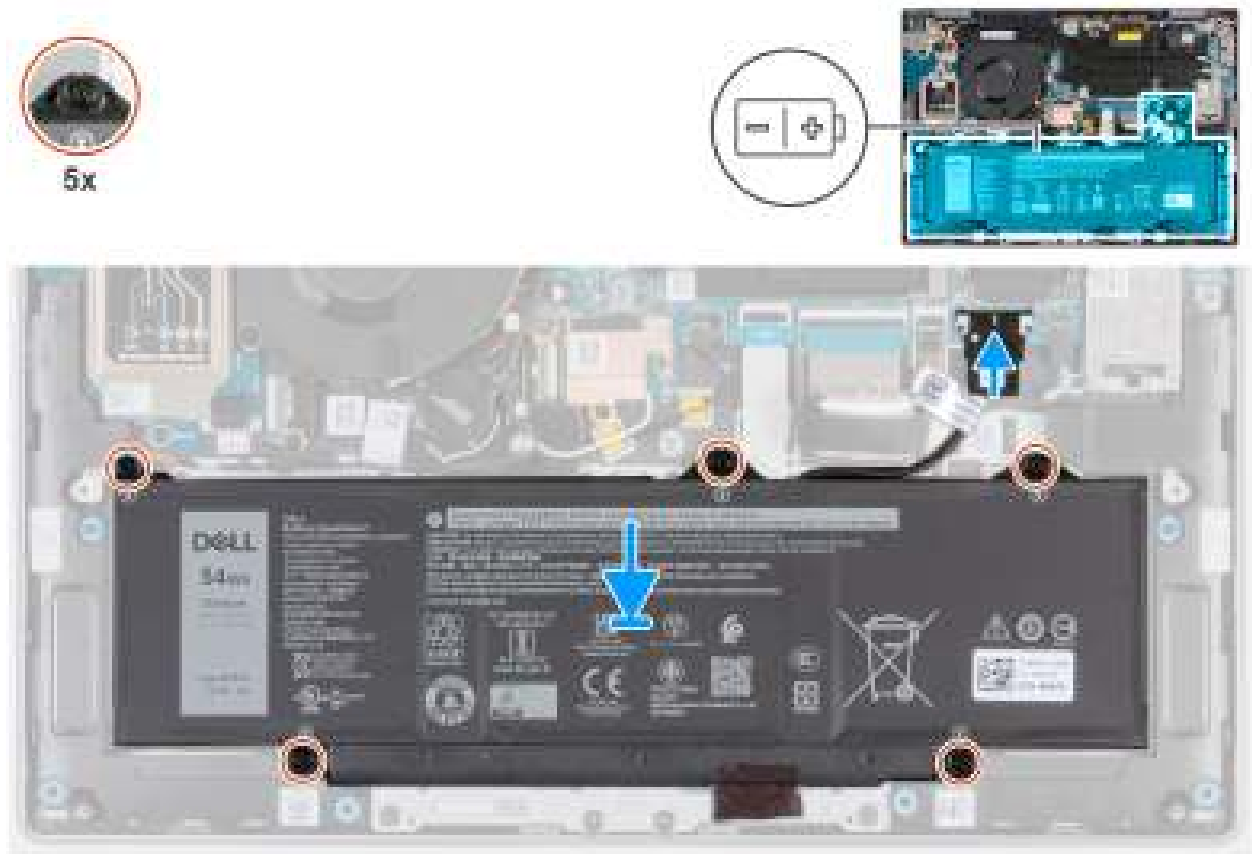
Afbeelding 40. De batterij plaatsen
