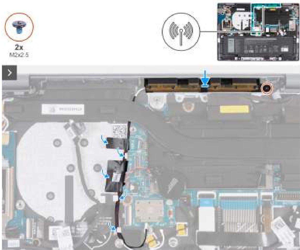
Afbeelding 69. De WLAN-antennemodule plaatsen (voor computers die worden geleverd met WWAN-ondersteuning)
