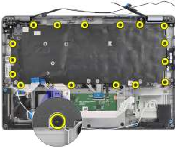
Afbeelding 80. Toetsenbordschroeven
