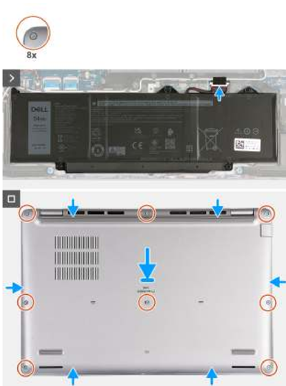
Afbeelding 13. De onderplaat plaatsen
