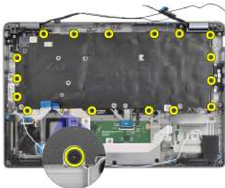
Afbeelding 82. Toetsenbordschroeven
