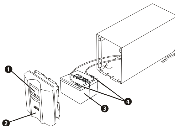
Toren SMT2200C, SMT2200IC, SMT3000C en SMT3000IC
