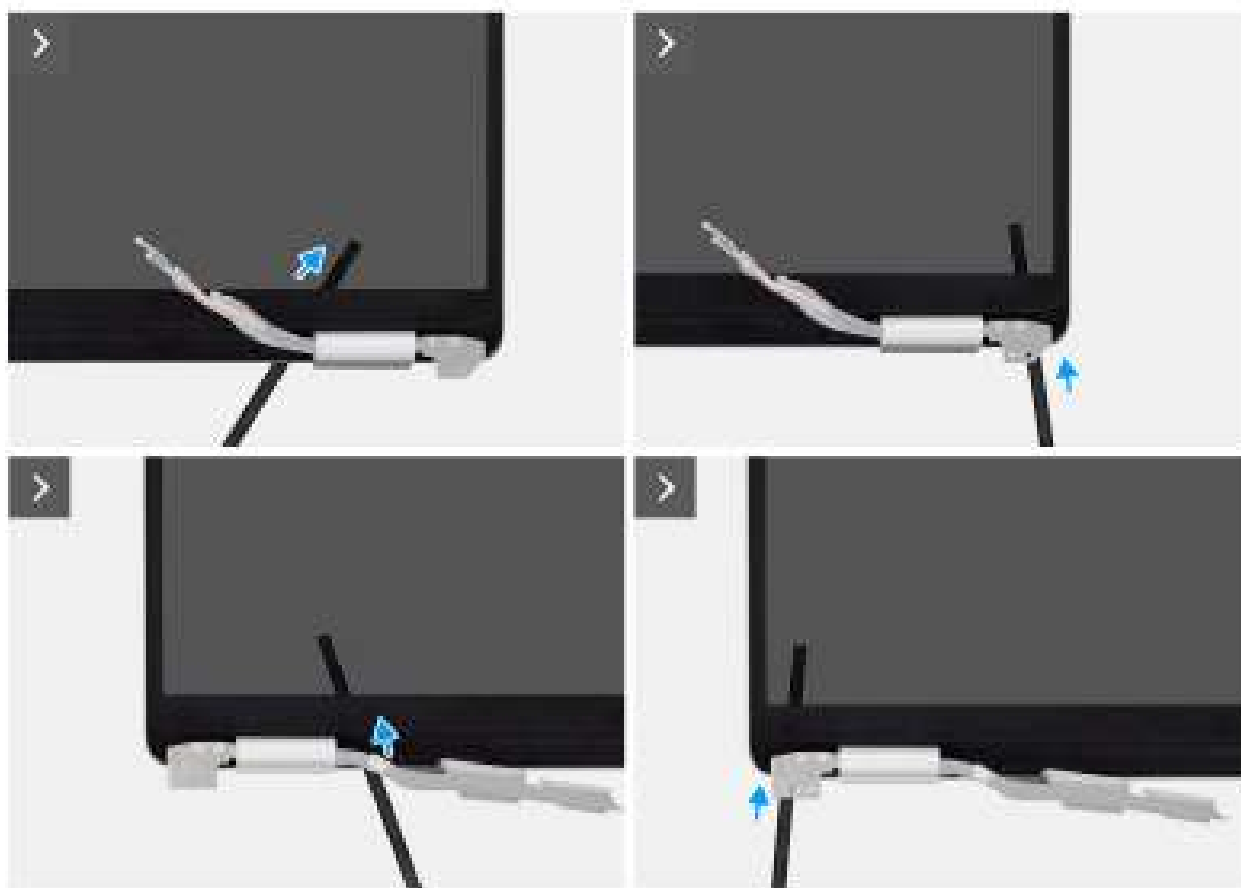
Figure 45. Levier sur la bordure le long des charnières
