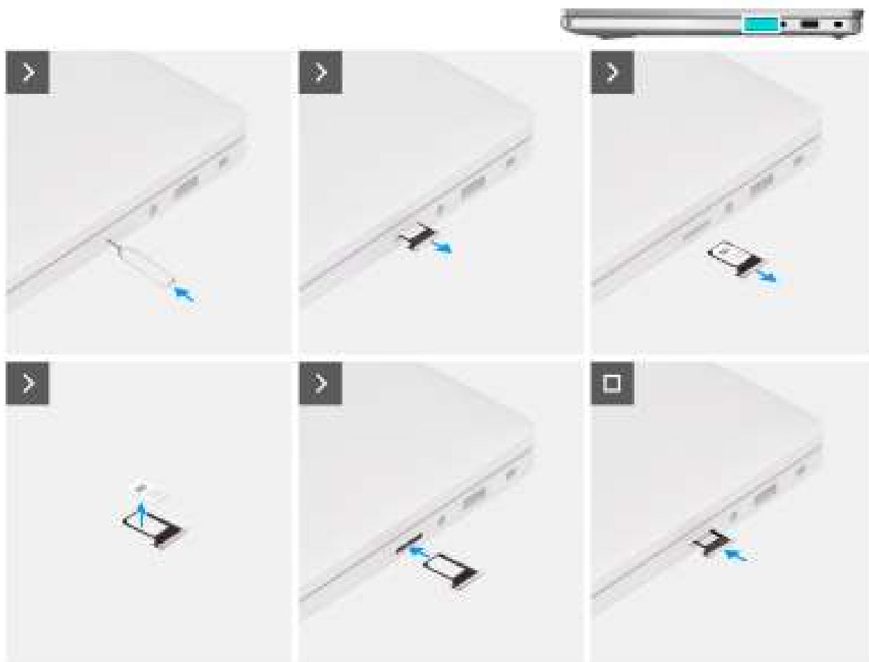
Figure 17. Retrait du plateau de carte SIM
