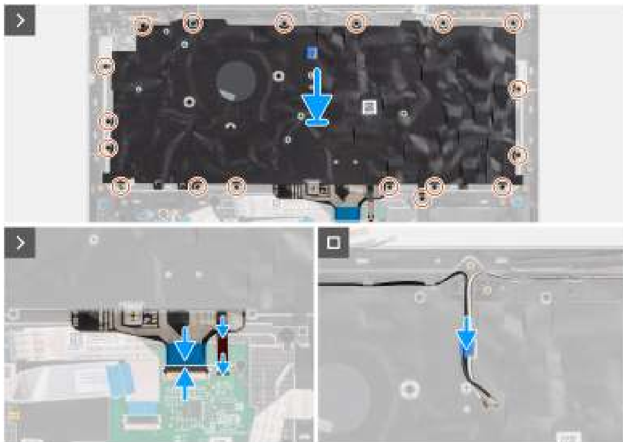
Figure 82. Installation du clavier
