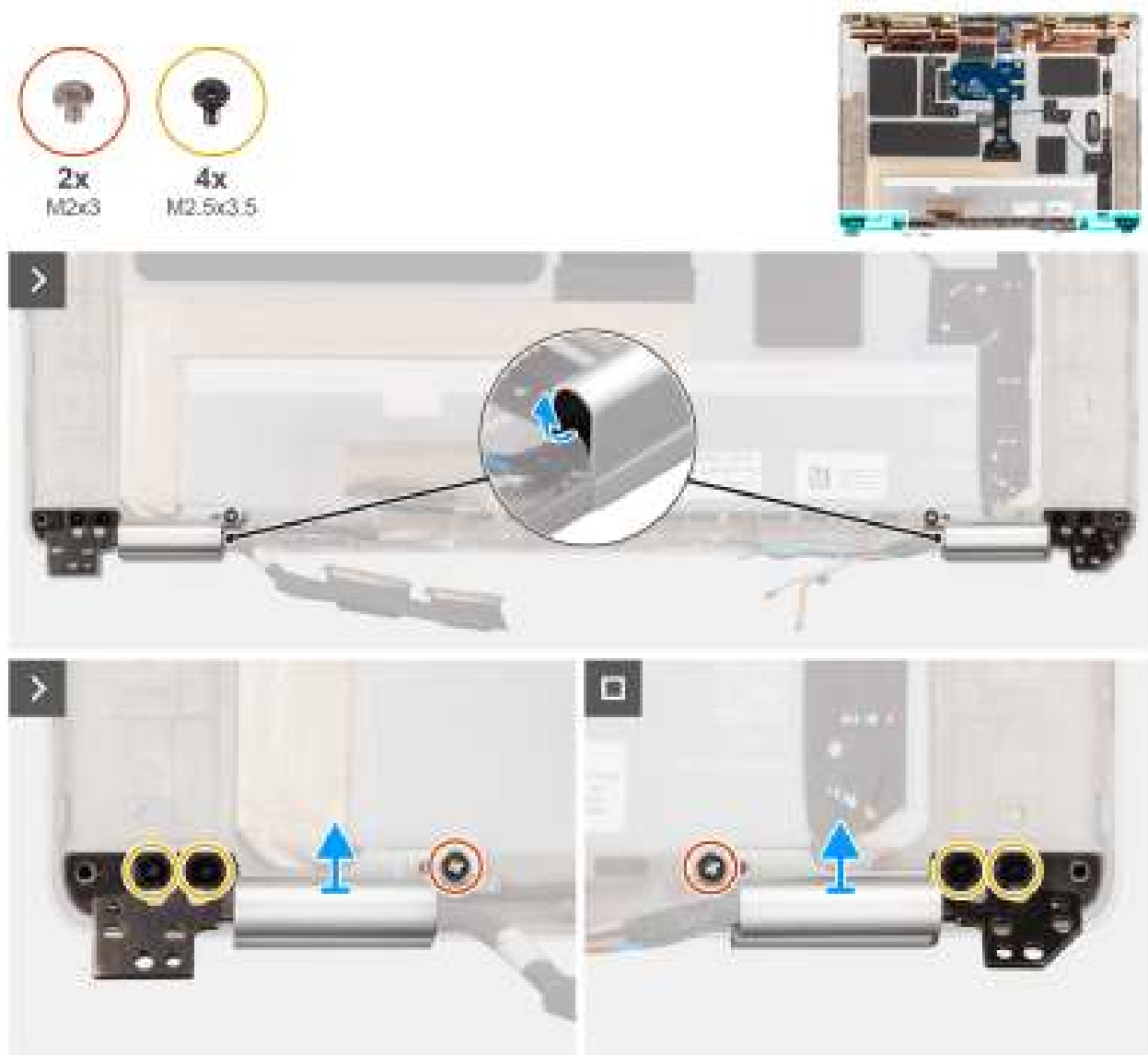
Figure 54. Retrait des charnières d'écran
