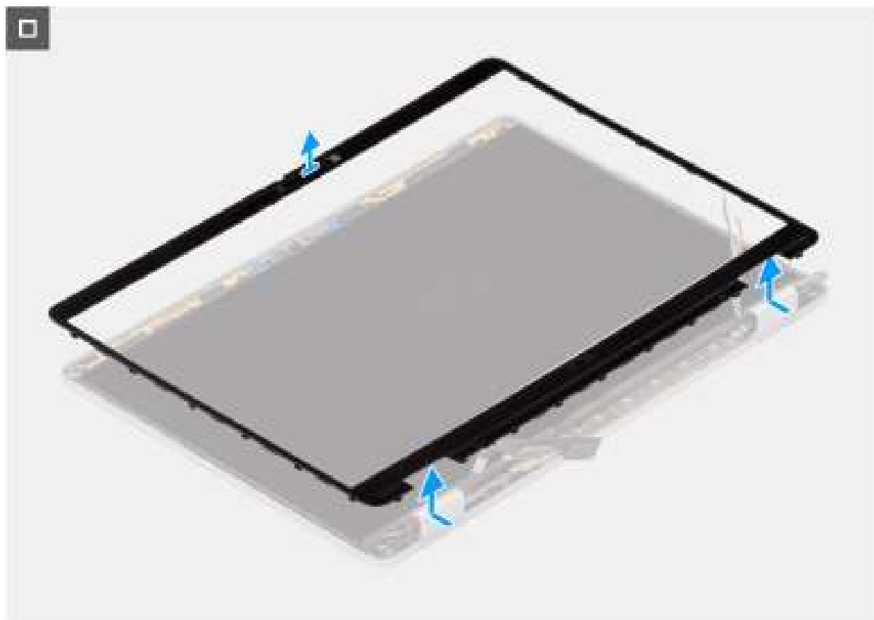
Figure 47. Retrait de la bordure d'écran
