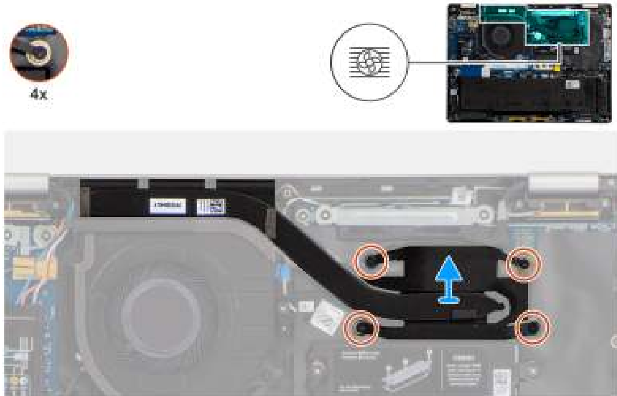
Figure 67. Retrait du dissipateur de chaleur
