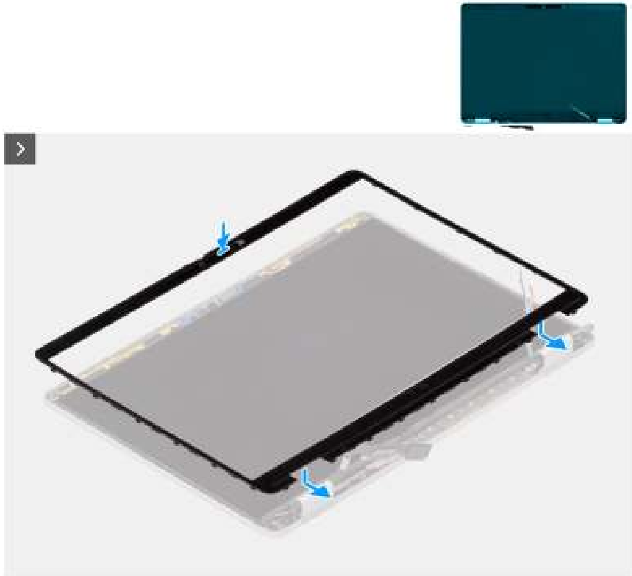
Figure 48. Installation de la bordure d'écran
