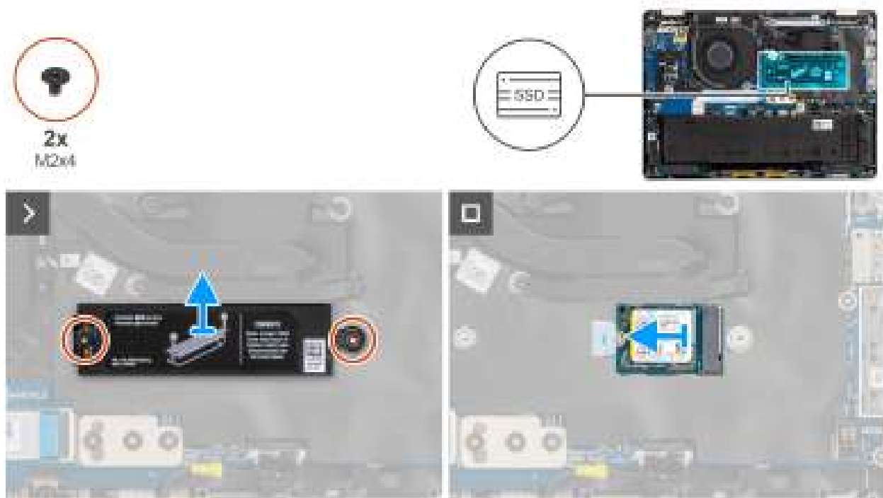
Figure 30. Retrait du disque SSD M.2 2230
