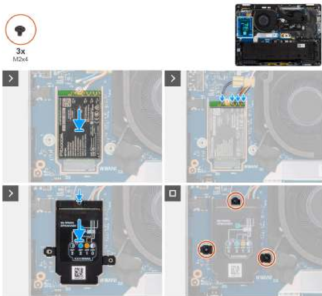
Figure 29. Installation de la carte WWAN
