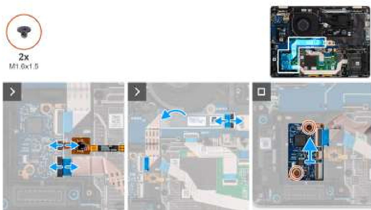
Figure 65. Retrait de la carte fille USH
