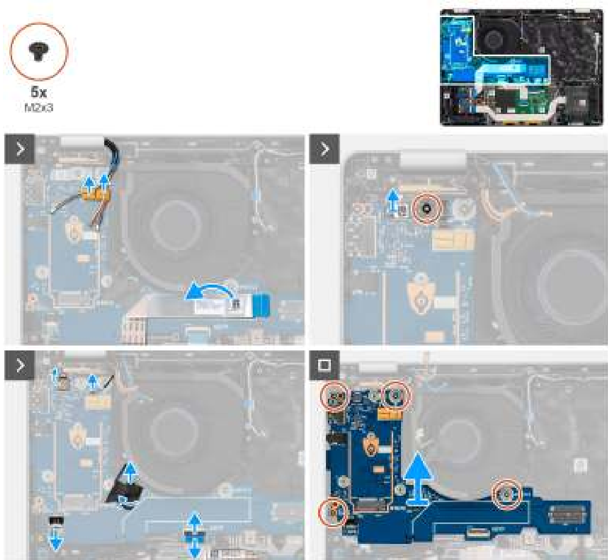
Figure 75. Retrait de la carte fille
