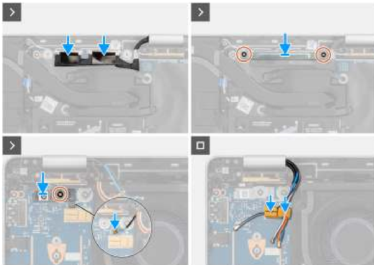
Figure 42. Alignement de l'assemblage d'écran avec l'assemblage du repose-poignets (2-en-1)
