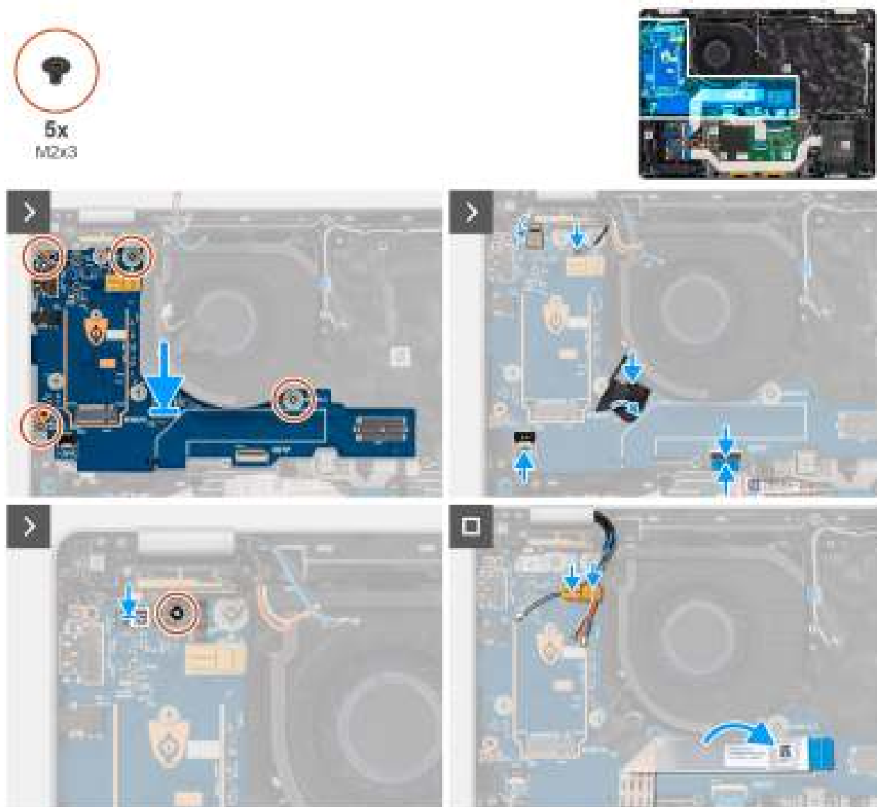
Figure 76. Installation de la carte d'E/S
