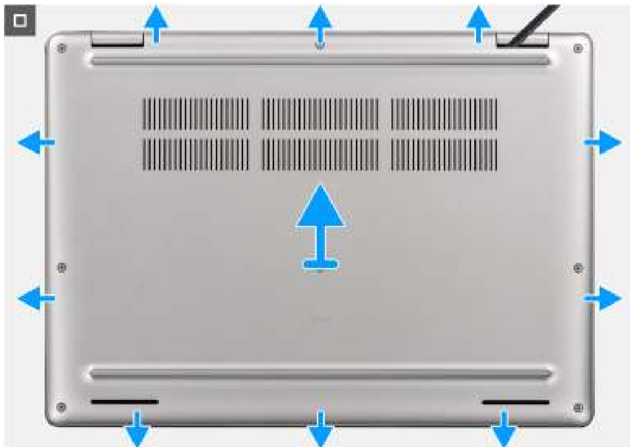
Figure 20. Retrait du cache de fond
