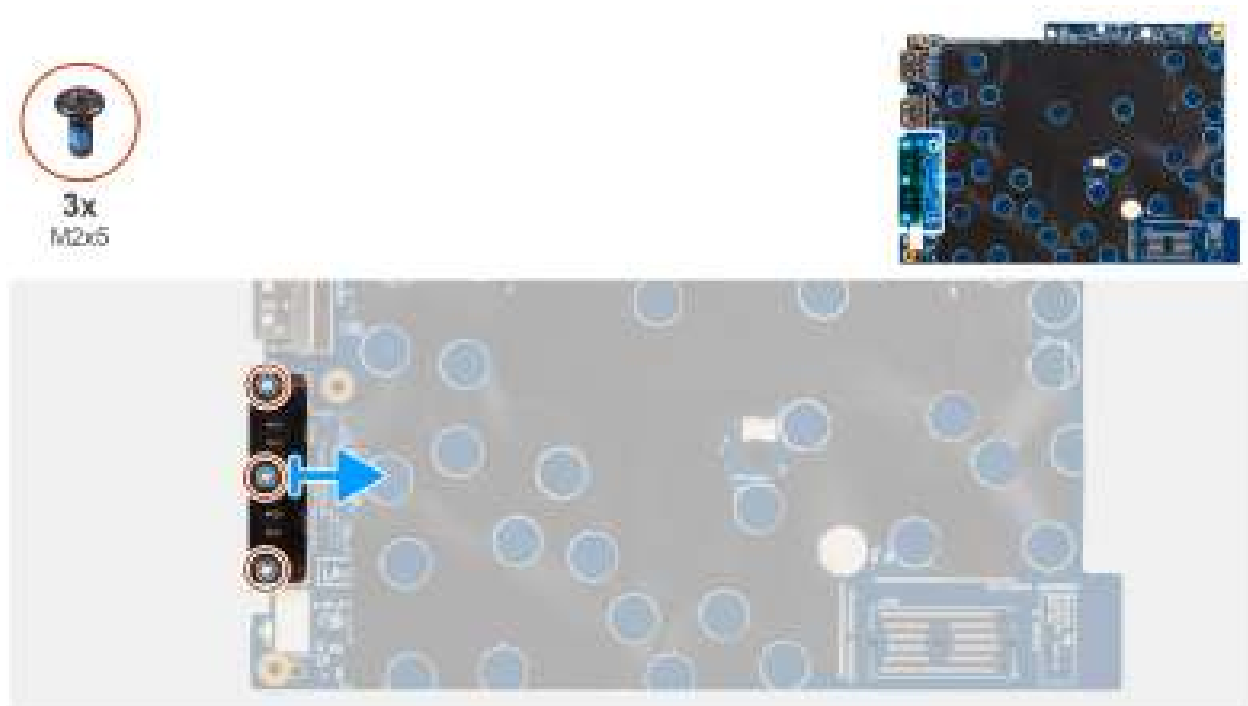
Figure 73. Retrait du module de connecteur USB-C
