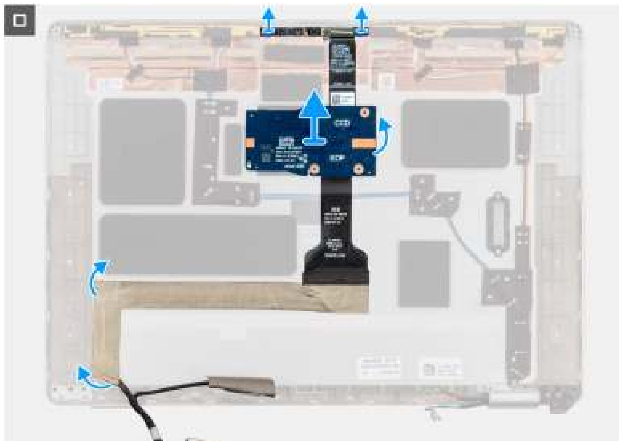
Figure 60. Retrait du câble de la caméra et de l'écran
