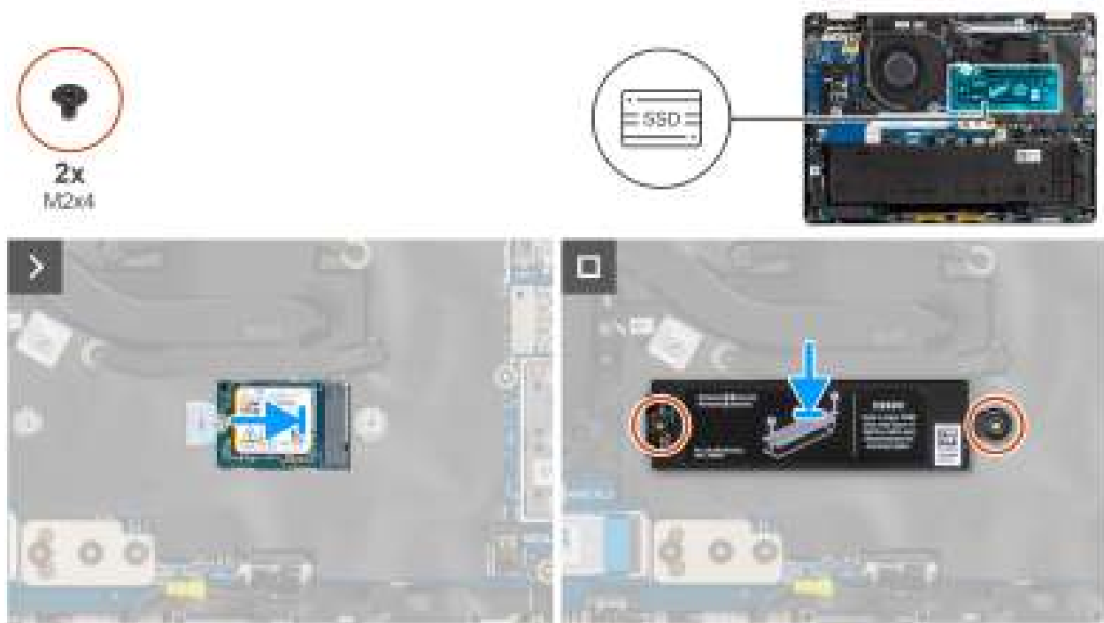
Figure 31. Installation du disque SSD M.2 2230
