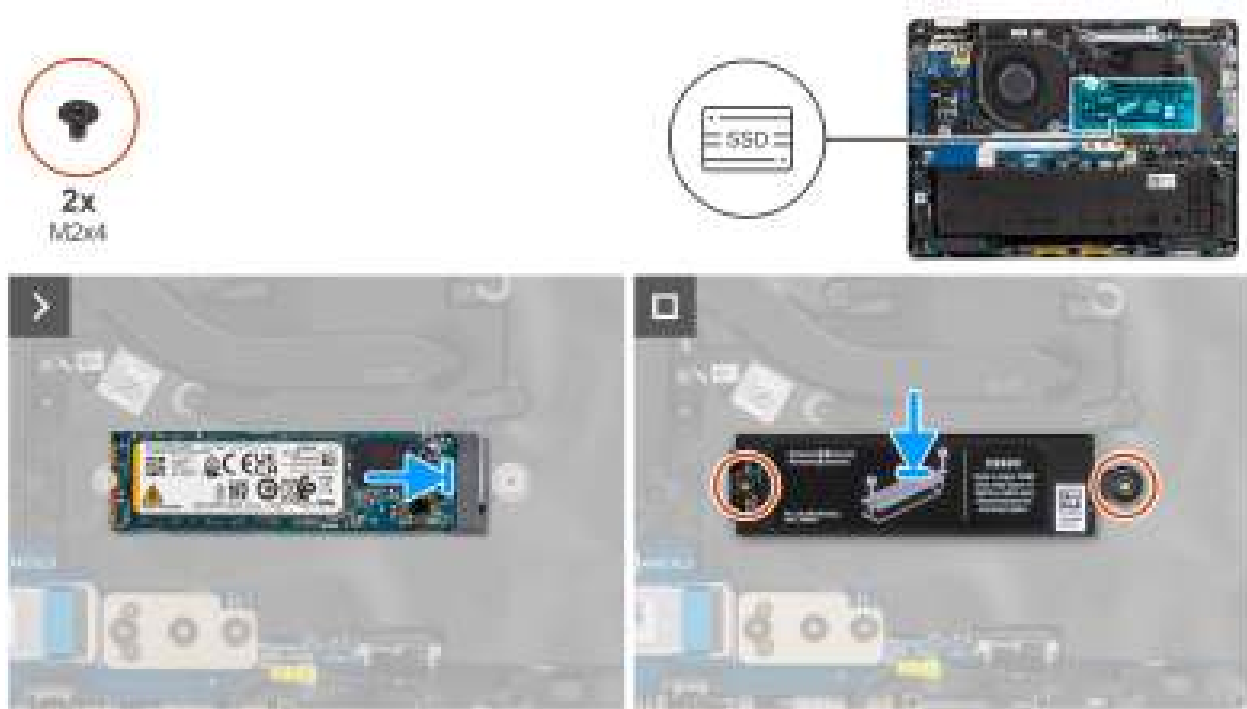
Figure 33. Installation du disque SSD M.2 2280
