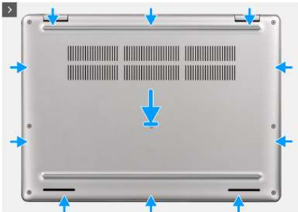
Figure 22. Installation du cache de fond
