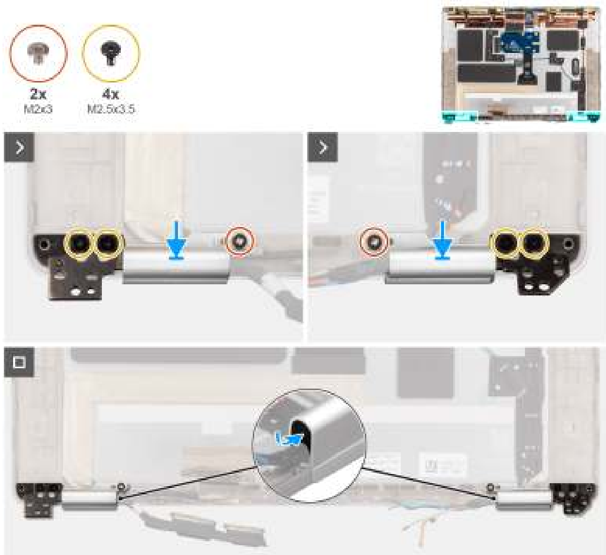
Figure 55. Installation des caches de charnière
