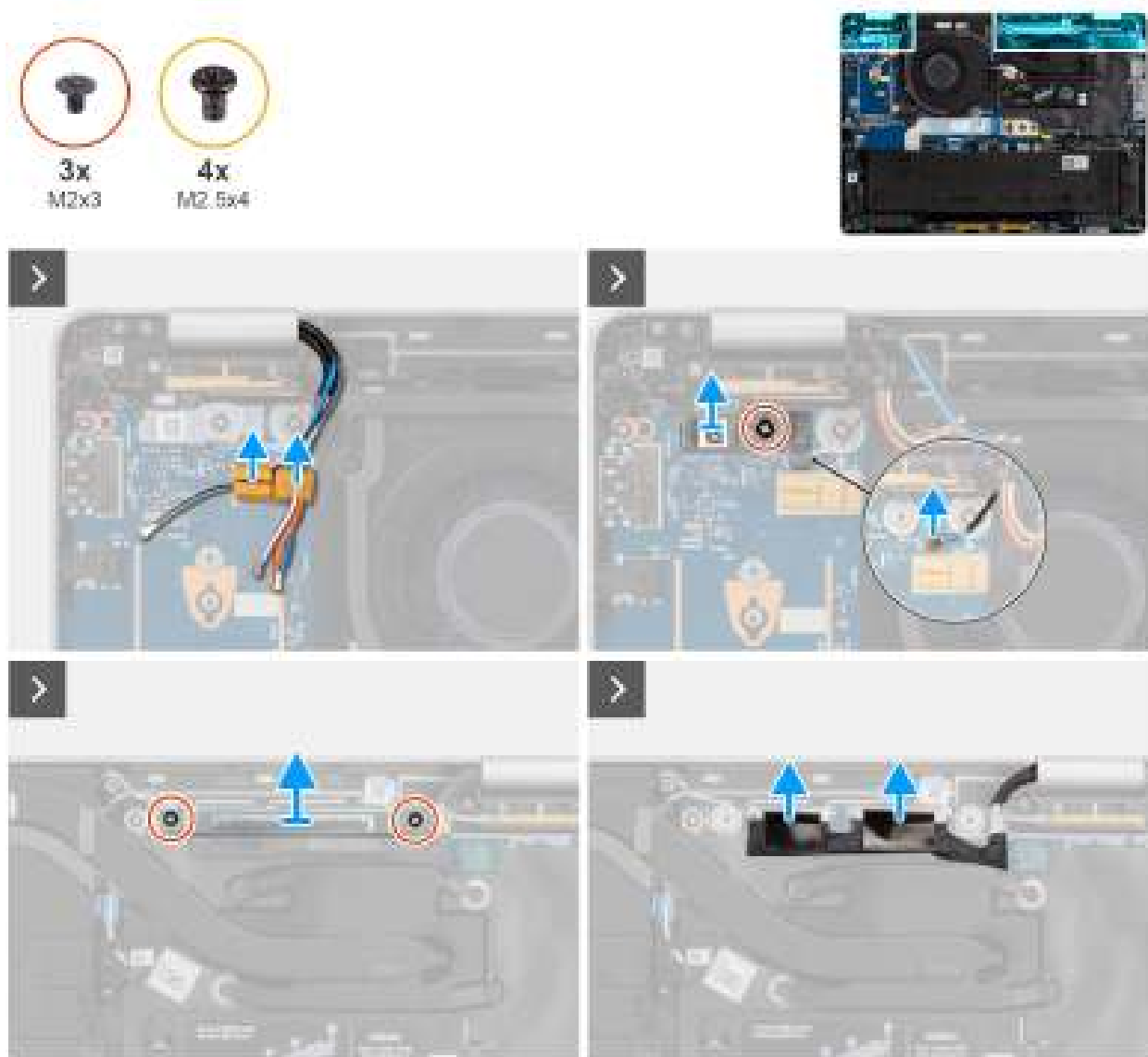
Figure 38. Retrait de l'assemblage d'écran
