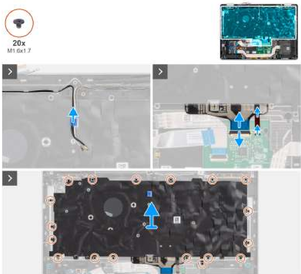
Figure 79. Retrait du clavier
