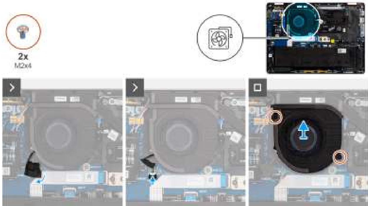
Figure 36. Retrait du ventilateur
