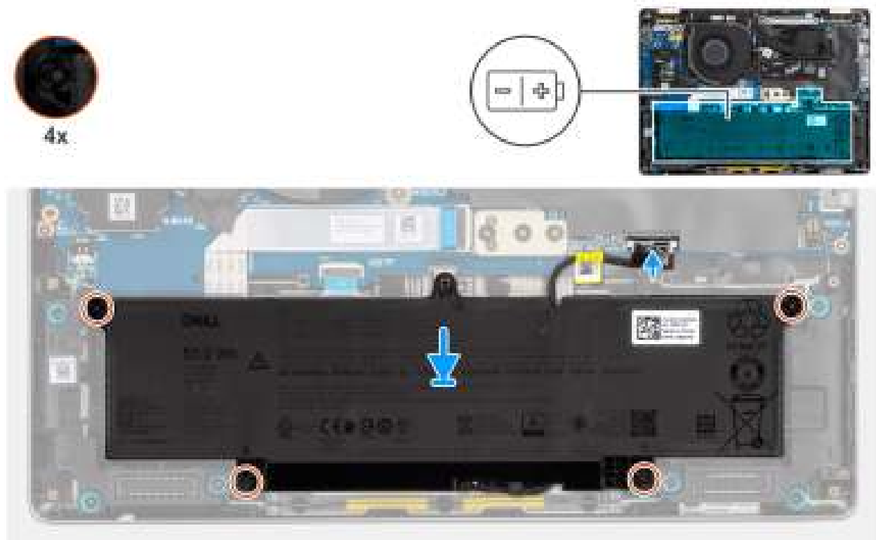
Figure 27. Installation de la batterie
