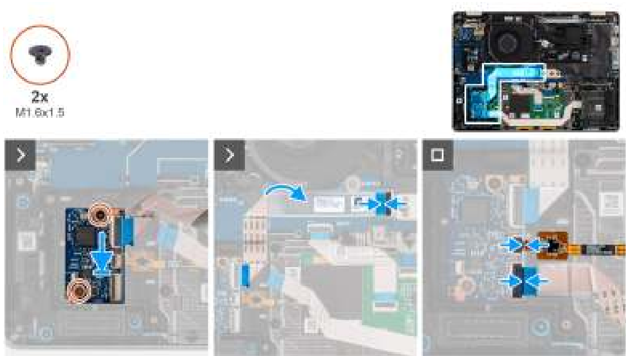
Figure 66. Installation de la carte fille USH
