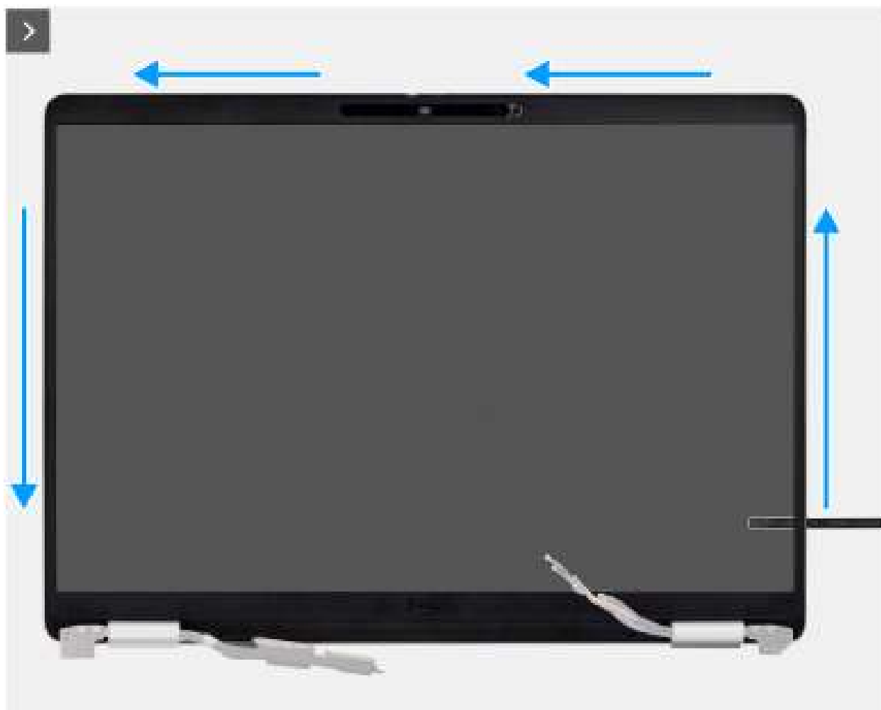
Figure 46. Levier sur la bordure le long des côtés
