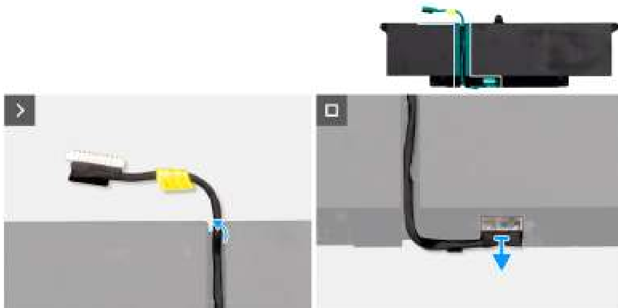
Figure 25. Retrait du câble de la batterie
