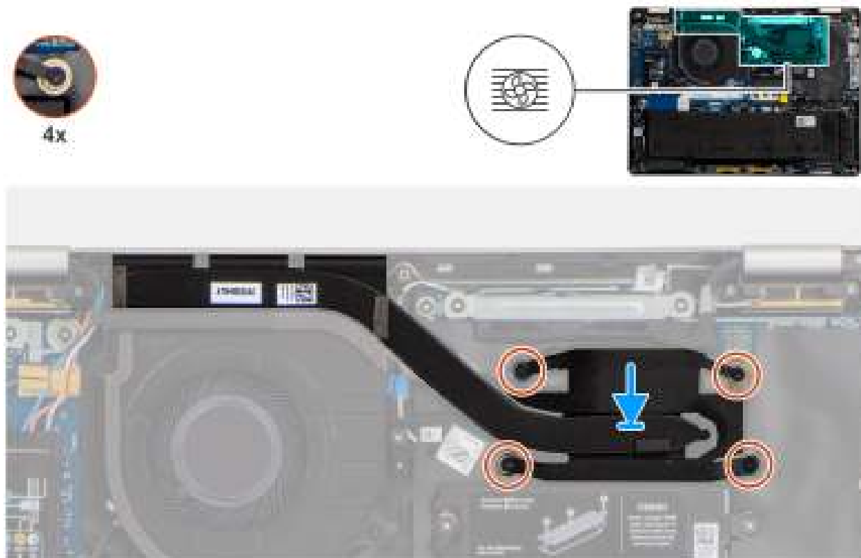
Figure 68. Installation du dissipateur de chaleur
