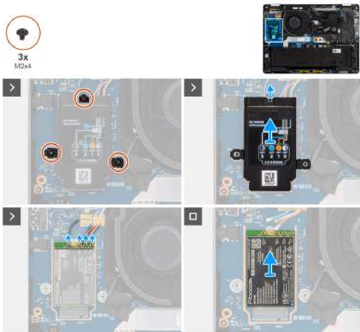
Figure 28. Retrait de la carte WWAN
