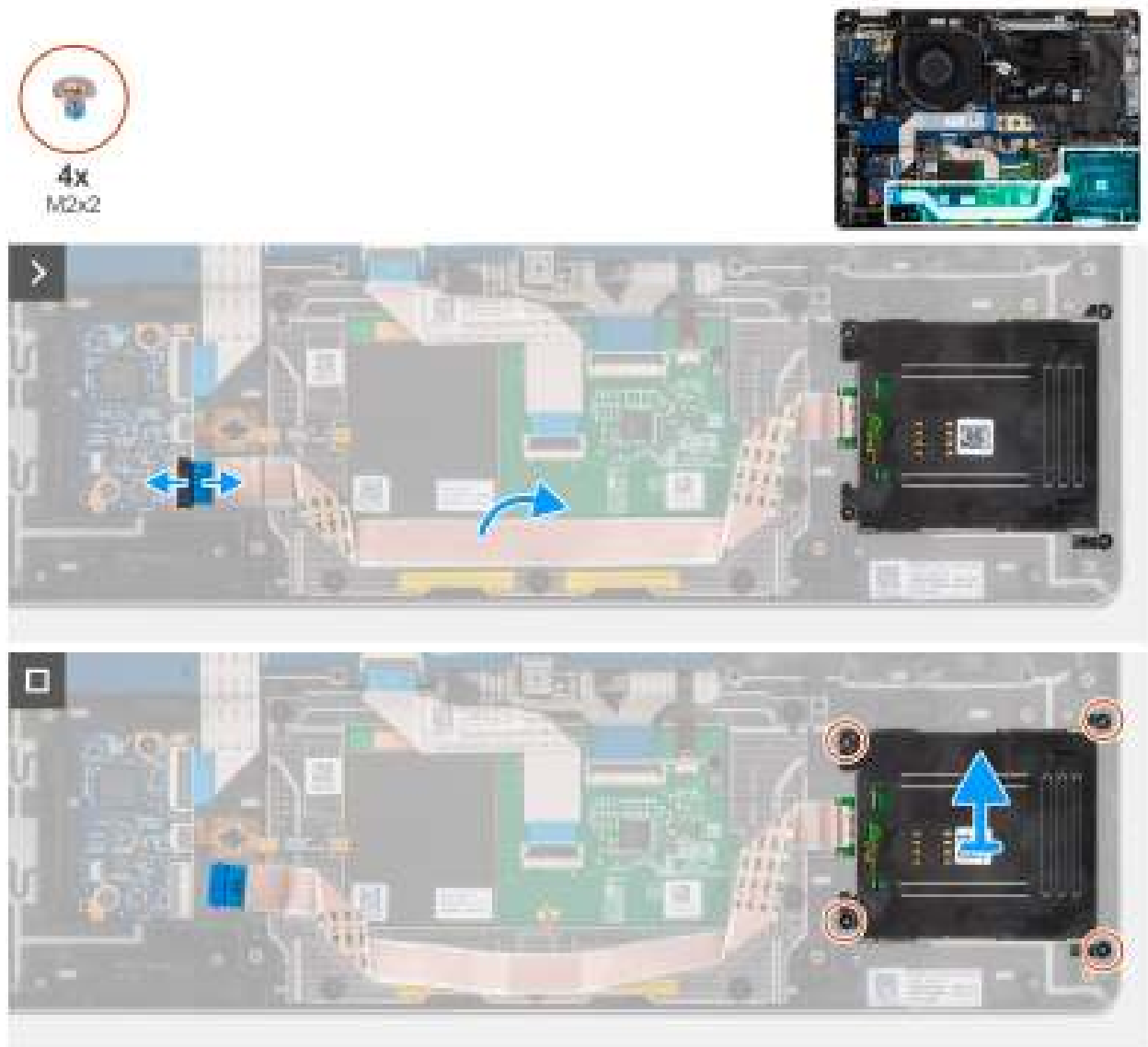
Figure 63. Retrait du lecteur de carte à puce
