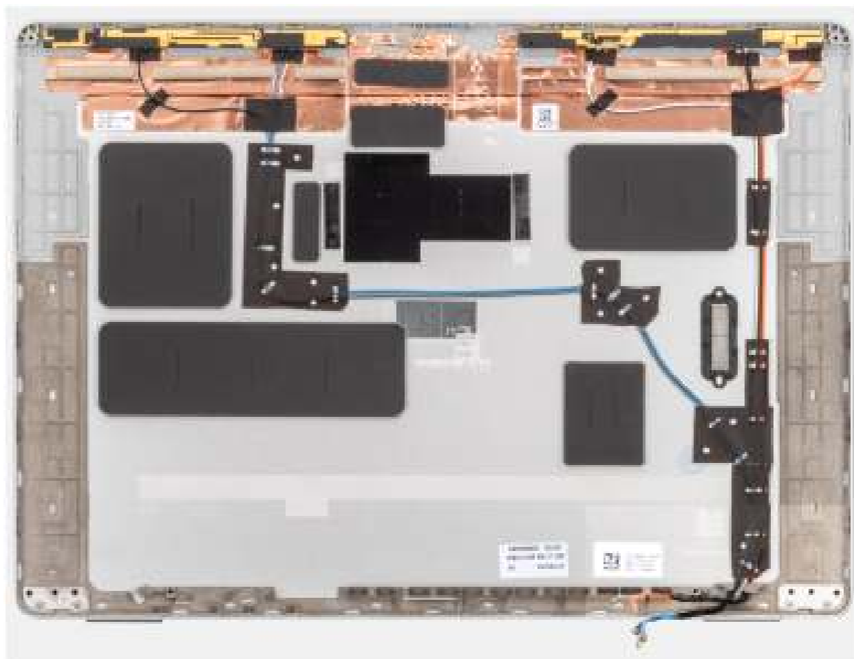
Figure 62. Retrait du capot arrière de l'assemblage d'écran
