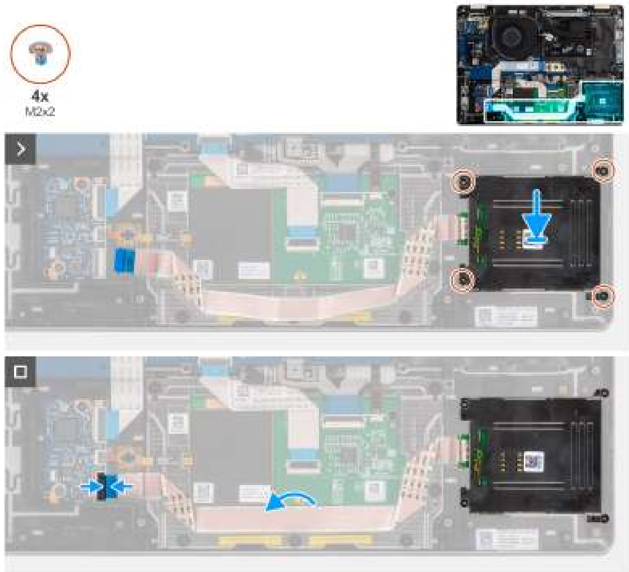
Figure 64. Installation du lecteur de carte à puce
