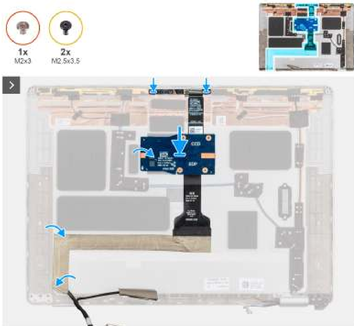
Figure 61. Installation du câble de la caméra et de l'écran
