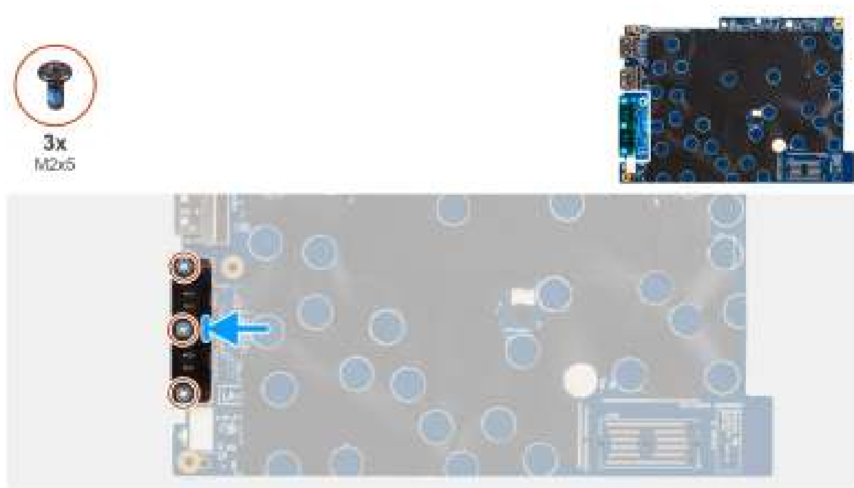
Figure 74. Installation du module de connecteur USB-C
