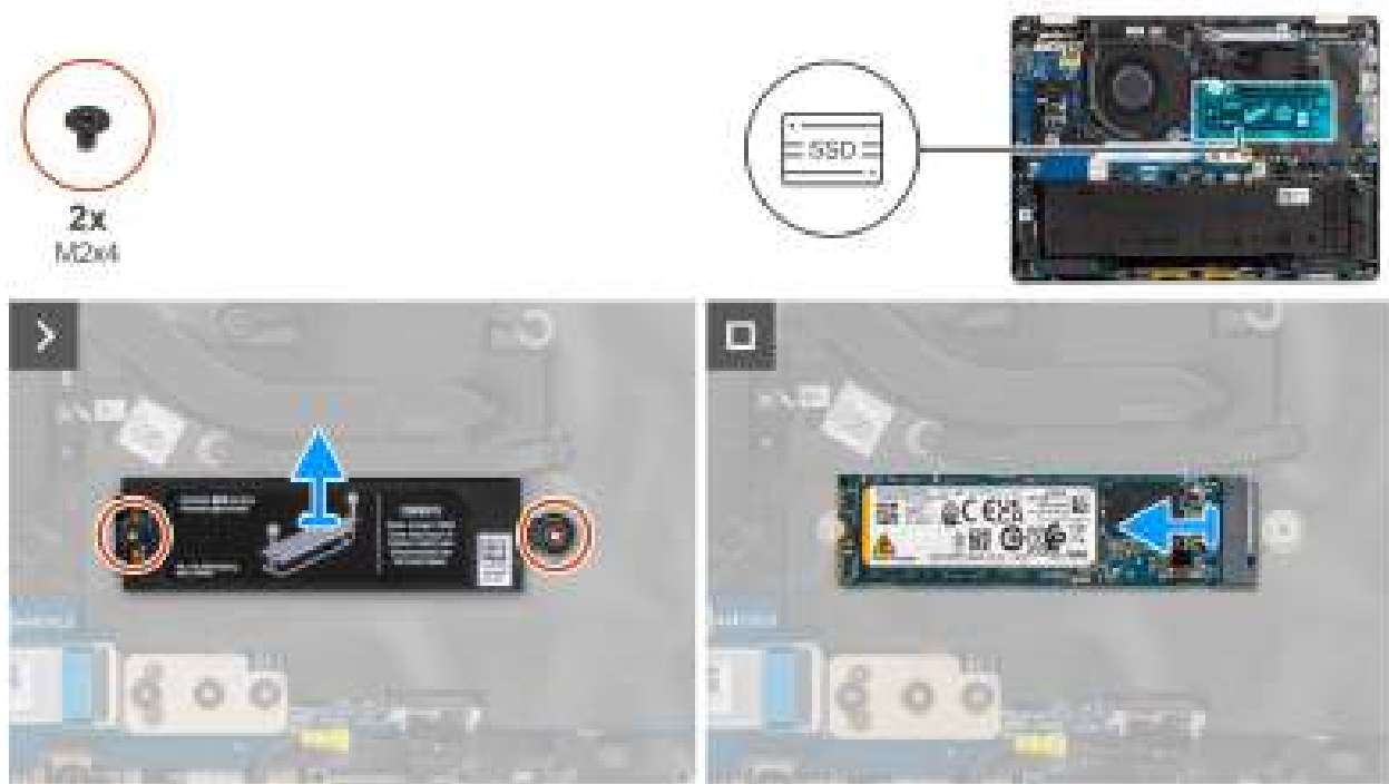
Figure 32. Retrait du disque SSD M.2 2280
