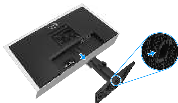
Schéma 20. Déposer le socle
