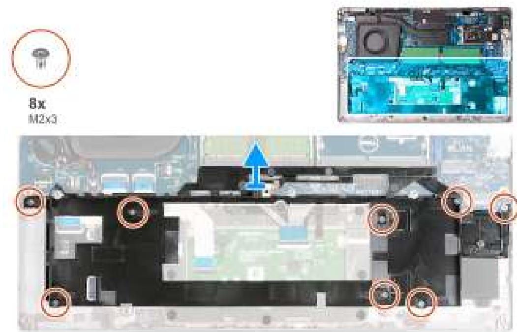
Figure 41. Retrait du cadre interne de l'assemblage
