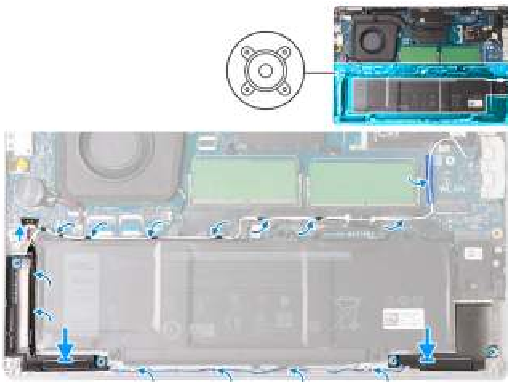
Figure 39. Installation des haut-parleurs
