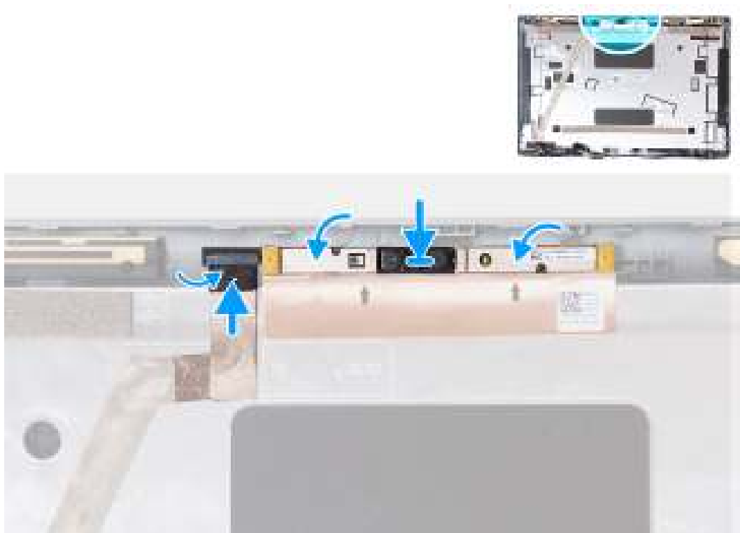
Figure 59. Installation du module de caméra
