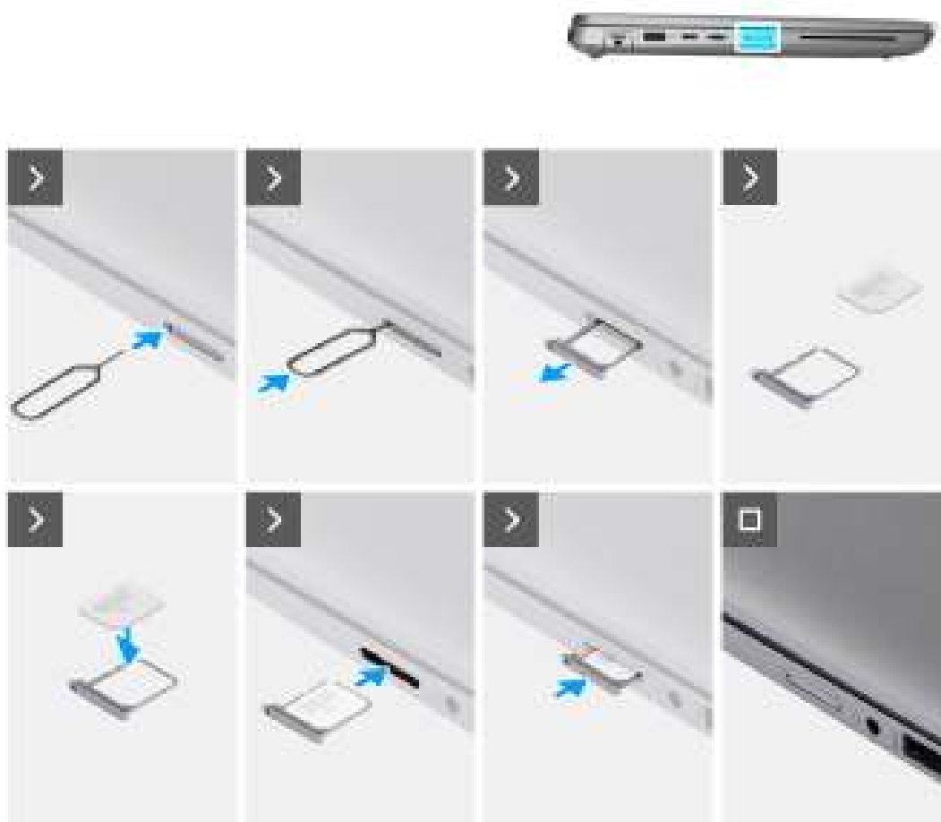
Figure 11. Installation du plateau de la carte SIM
