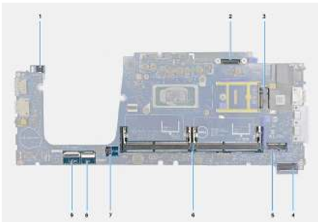
Figure 71. Connecteurs de la carte système
