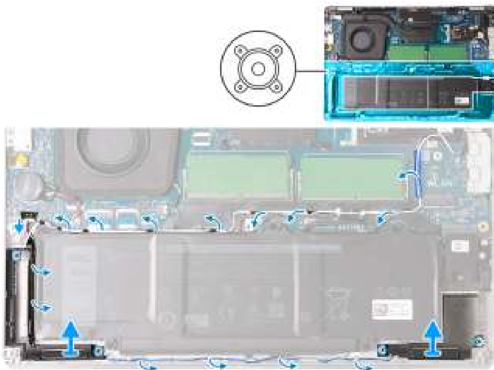
Figure 38. Retrait des haut-parleurs
