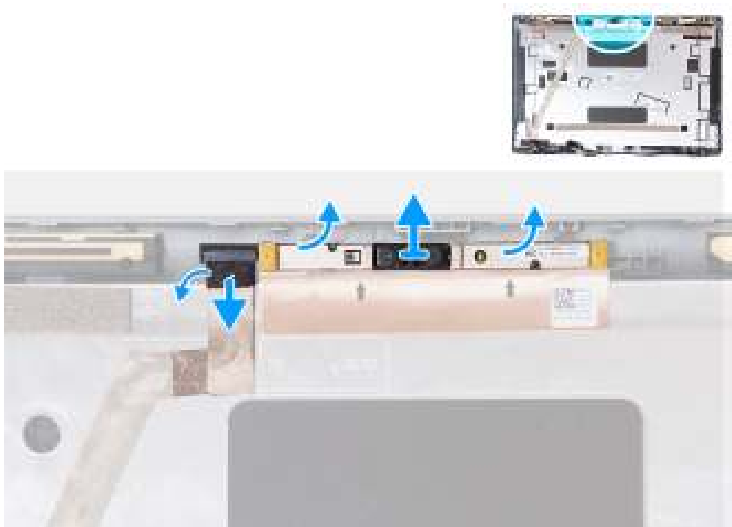
Figure 58. Retrait du module de caméra
