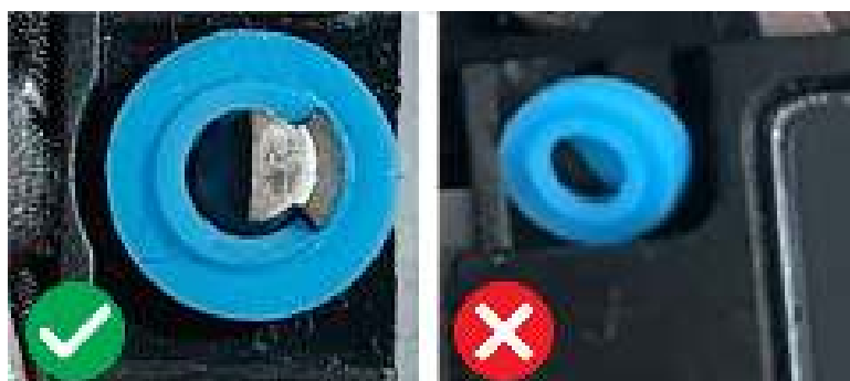
Figure 40. Positionnement des passe-câbles en caoutchouc
