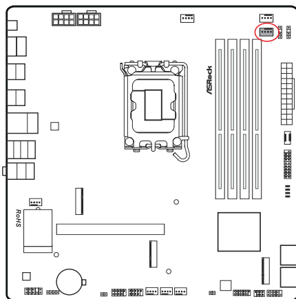
AIO_PUMP
